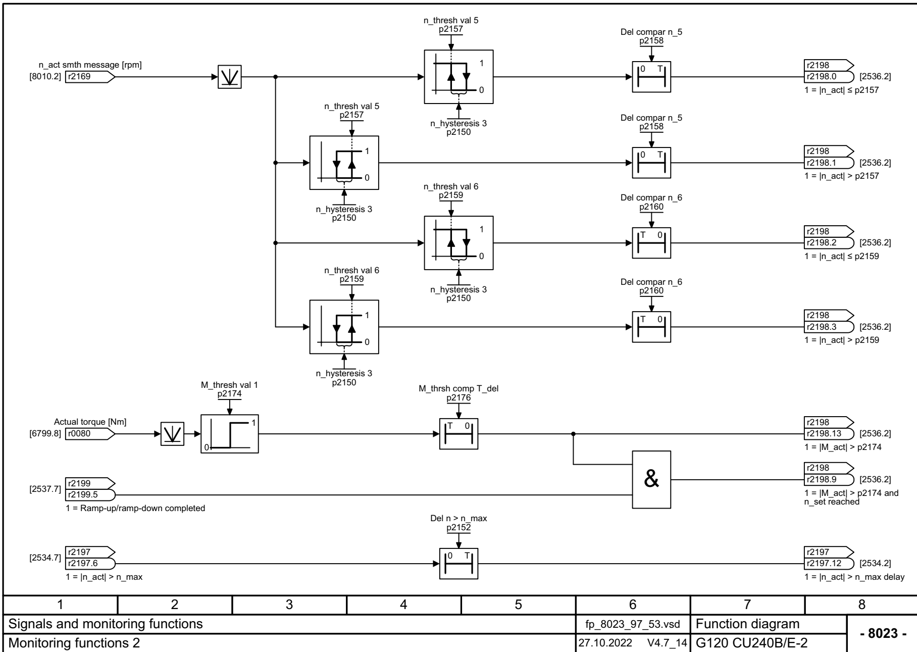
图 3-181 8023 - 监控功能 2
