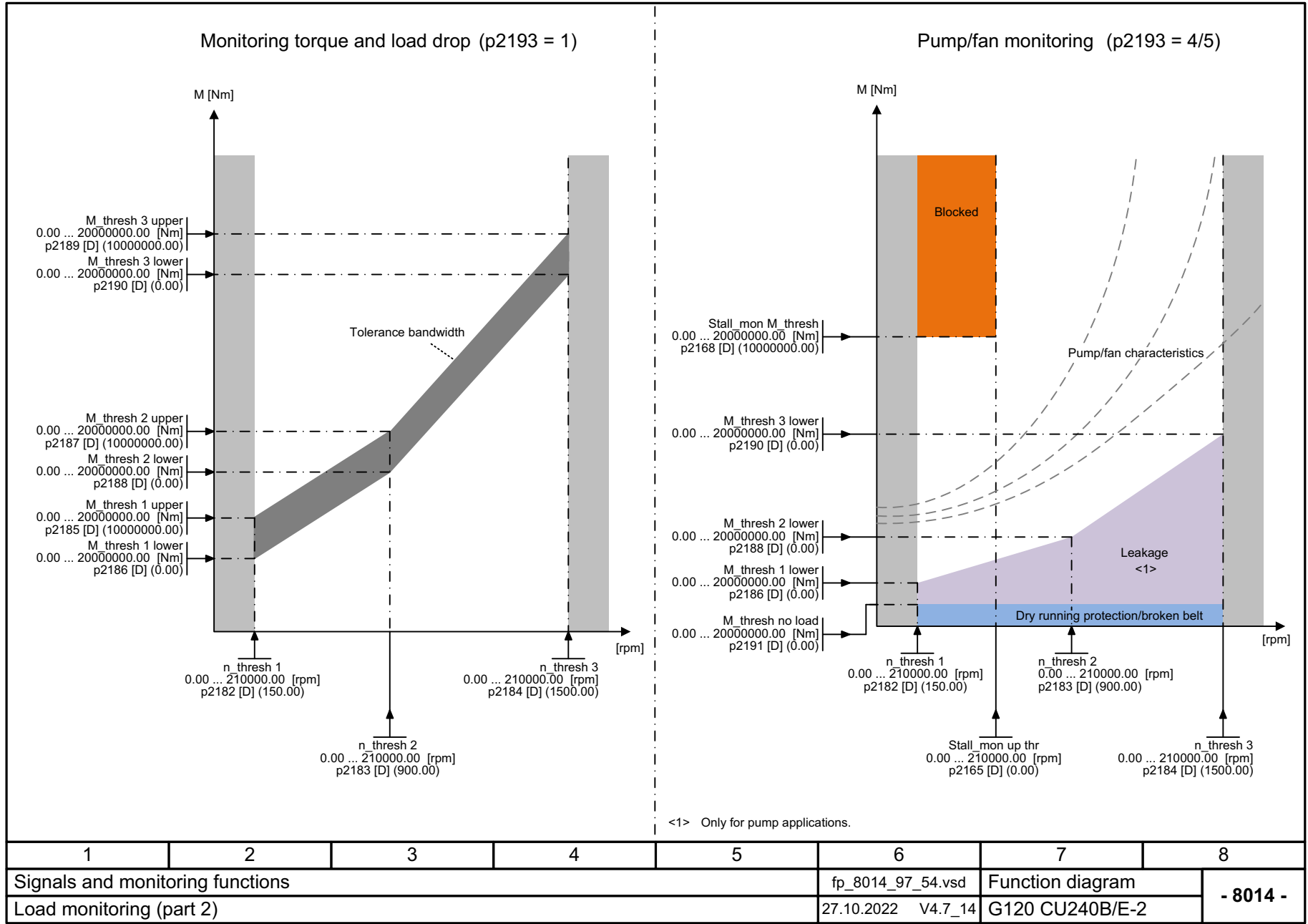
图 3-174 8014 - 负载监控 (第 2 部分)
