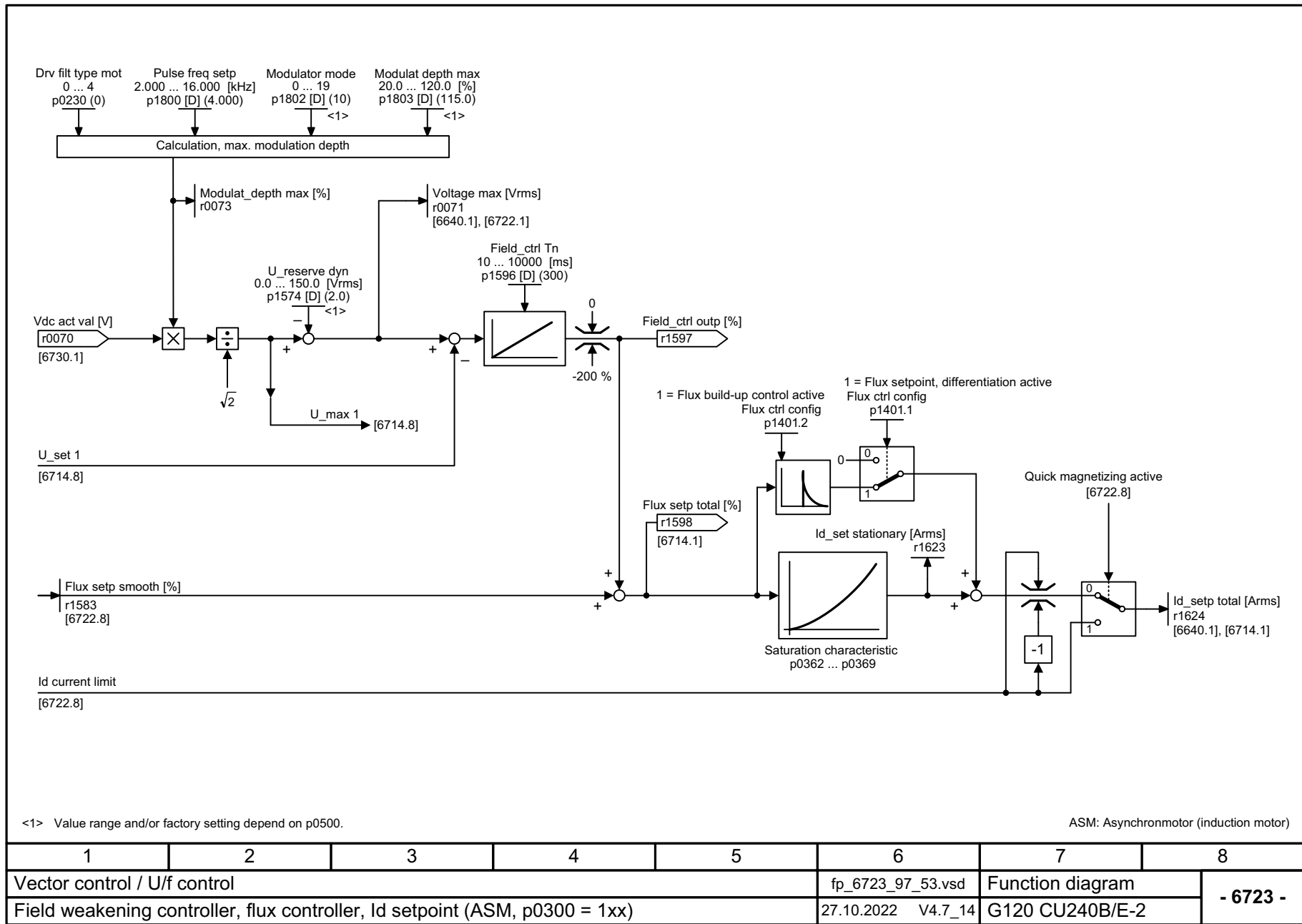
图 3-110 6723 - 弱磁调节器，磁通调节器，Id 设定值 (ASM, p0300 = 1)
