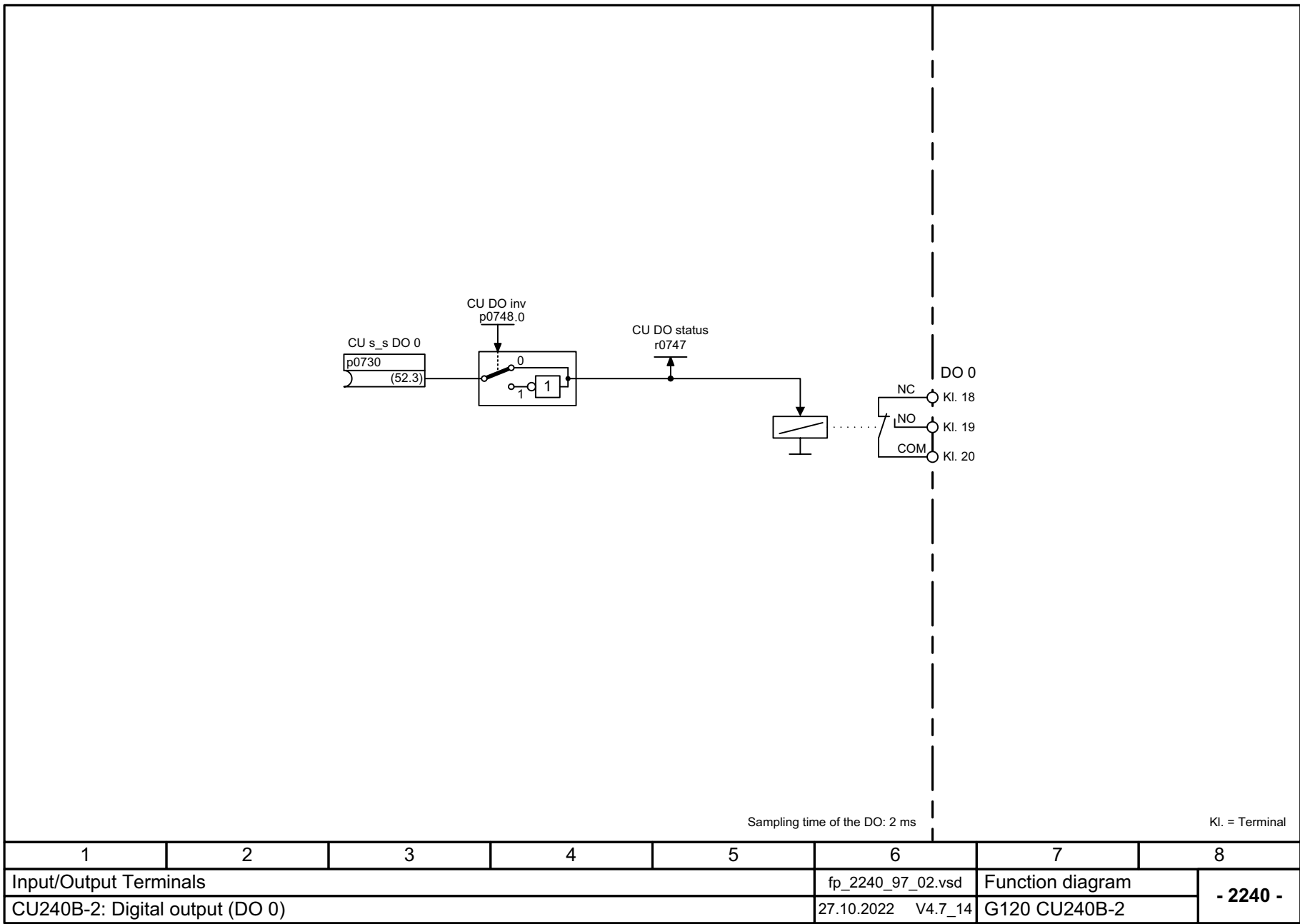
图 3-9 2240 - CU240B-2: 数字量输出端 (DO 0) SINAMICS G120 控制单元 CU240B-2/CU240E-2 参数手册, 2023/02, A5E3889529
