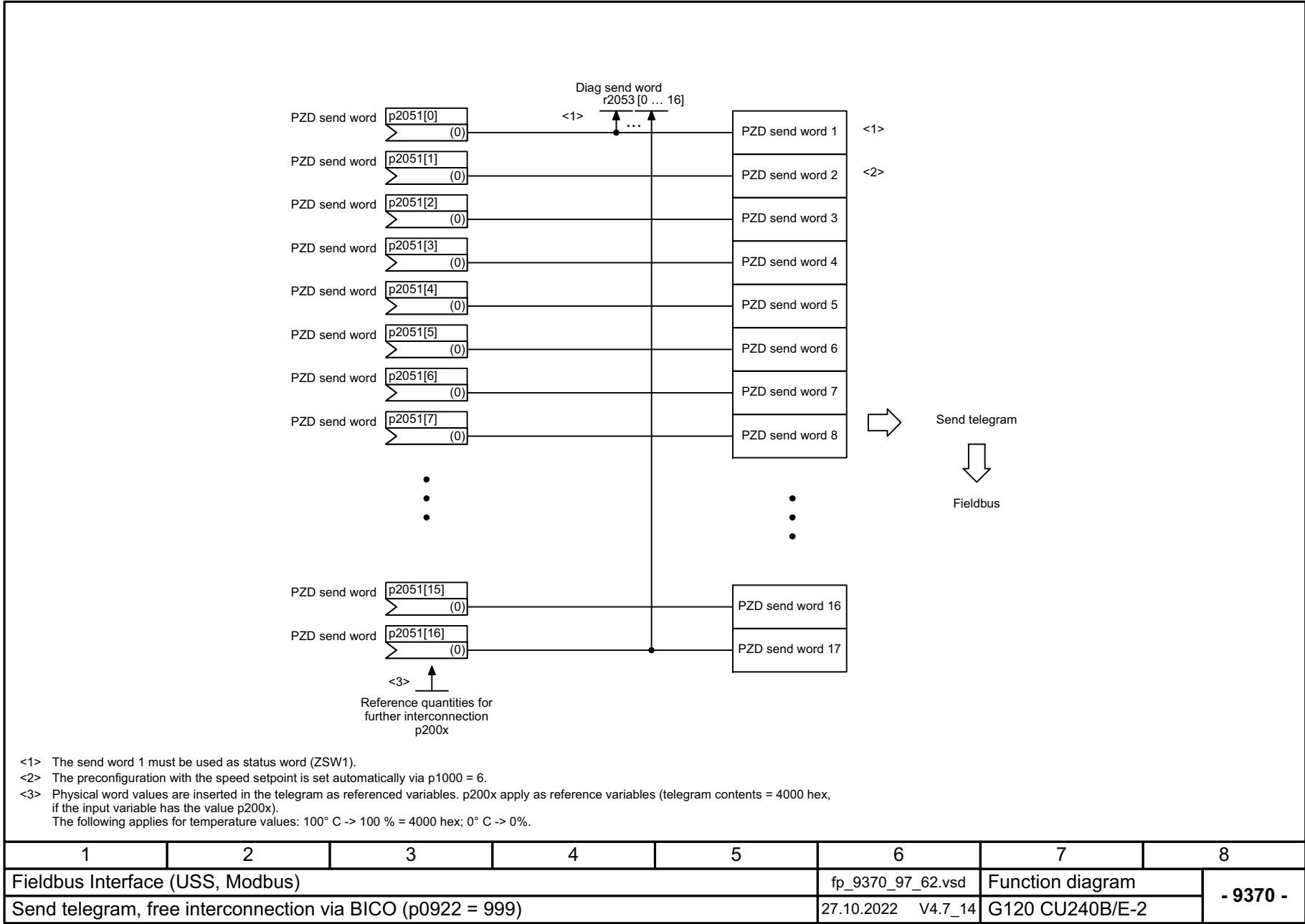
图 3-40 9370 - 通过 BICO 自由互联发送报文 (p0922 = 999)
