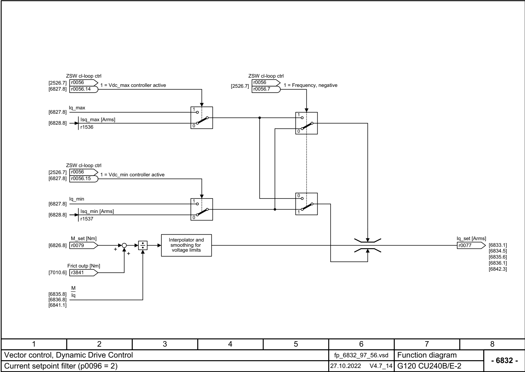
图 3-131 6832 - 电流设定值滤波器 (p0096 = 2)
