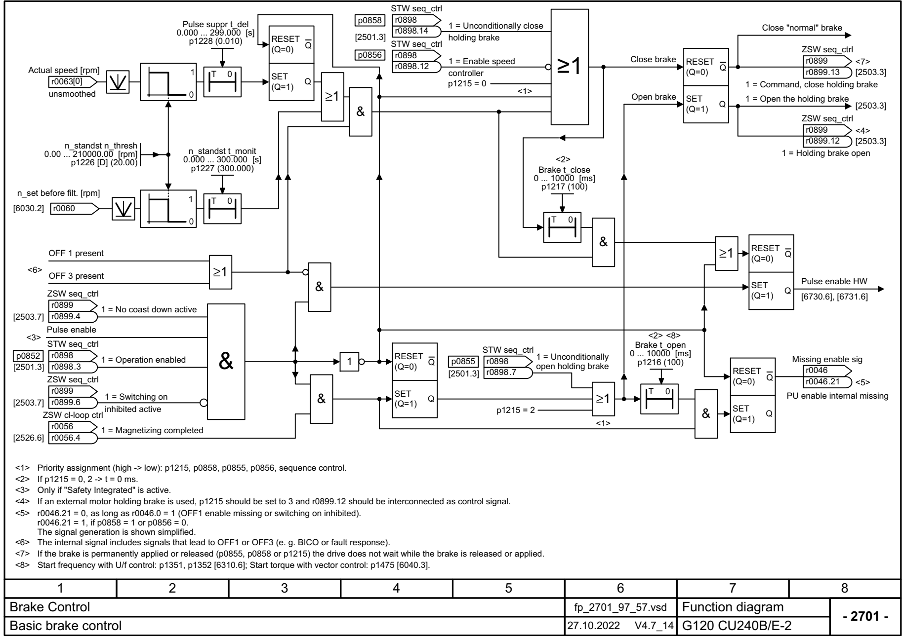
图 3-60 2701 - 简单制动控制
