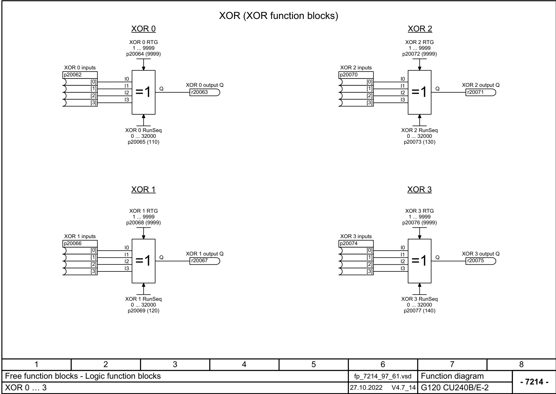
图 3-147 7214 - XOR 0 ... 3
