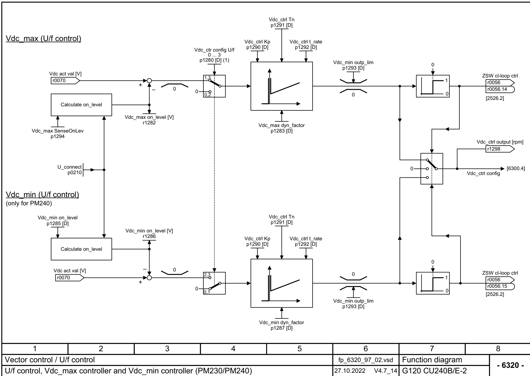
图 3-100 6320 - V/f 控制、Vdc_max 控制器和 Vdc_min 控制器 (PM230/PM240)
