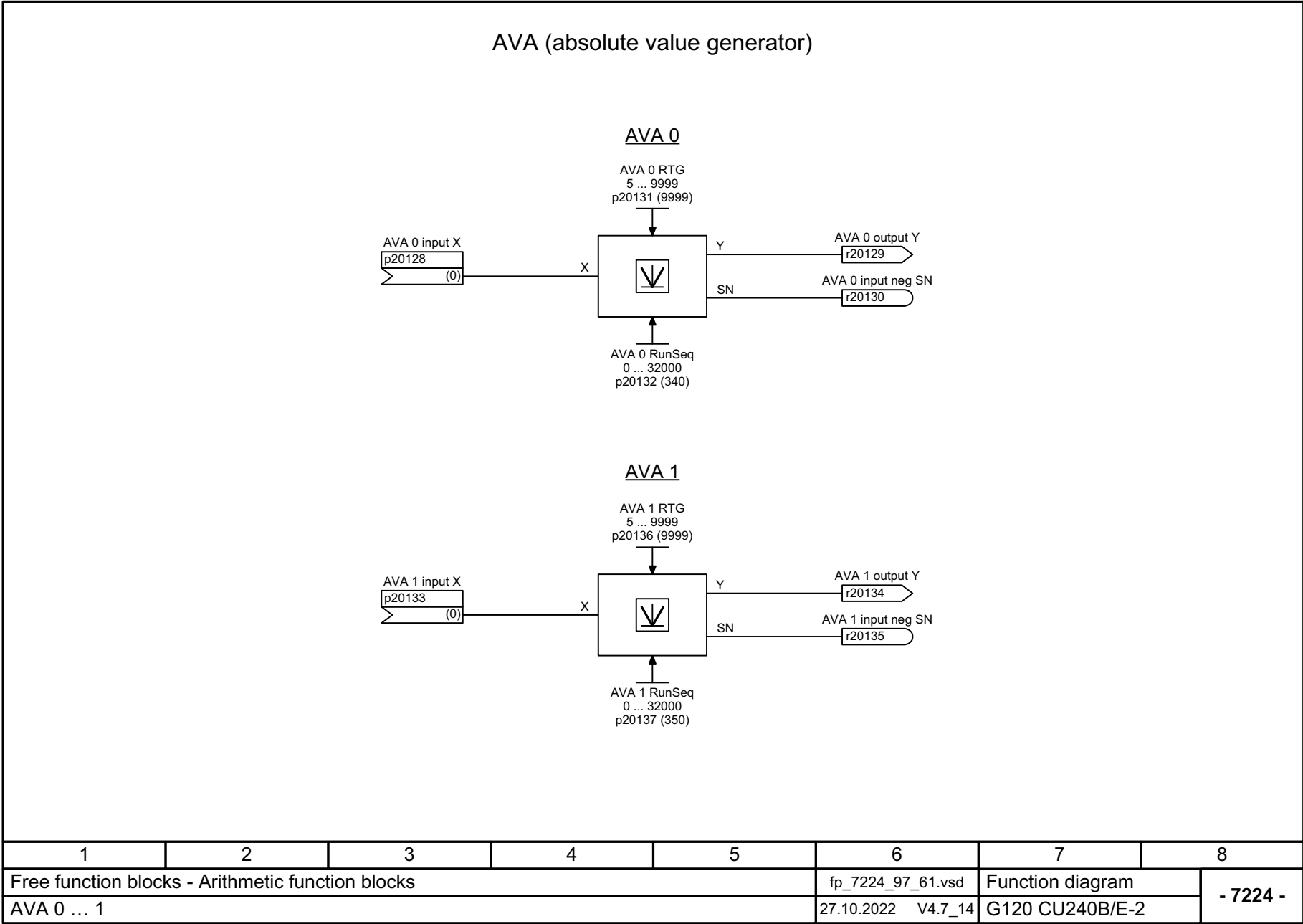
图 3-151 7224 - AVA 0 ... 1
