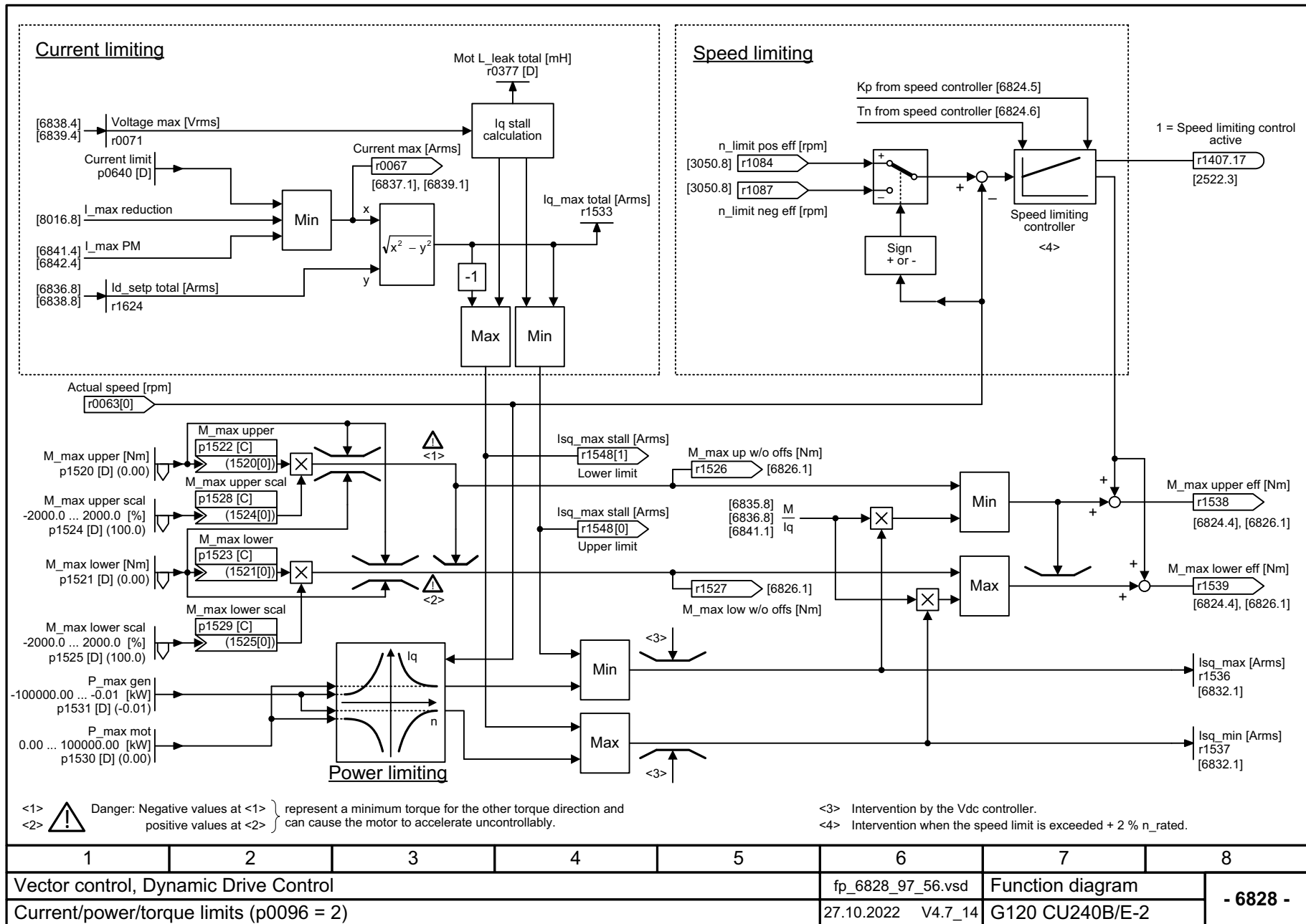
图 3-130 6828 - 电流极限 / 功率极限 / 转矩极限 (p0096 = 2)
