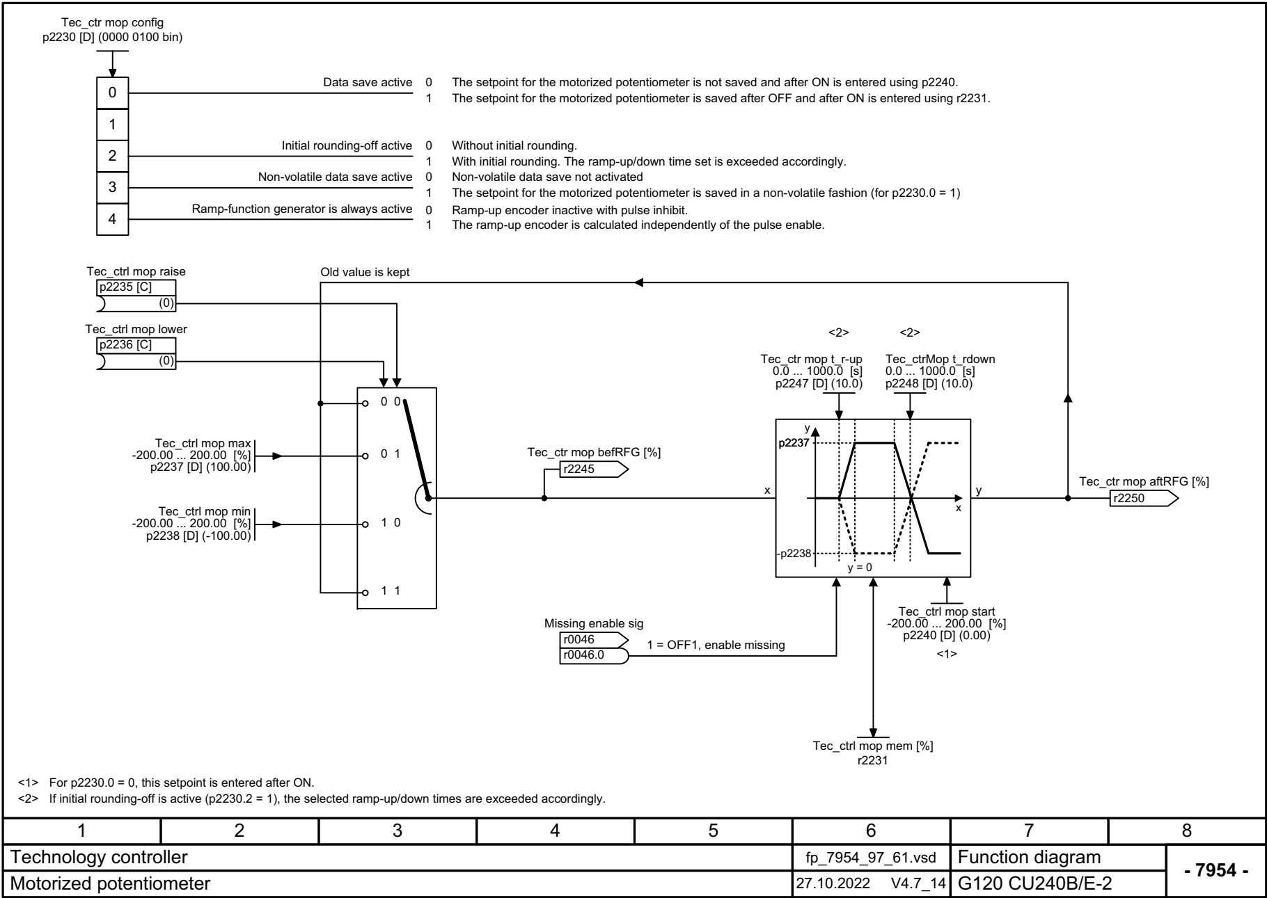
图 3-166 7954 - 电动电位计
