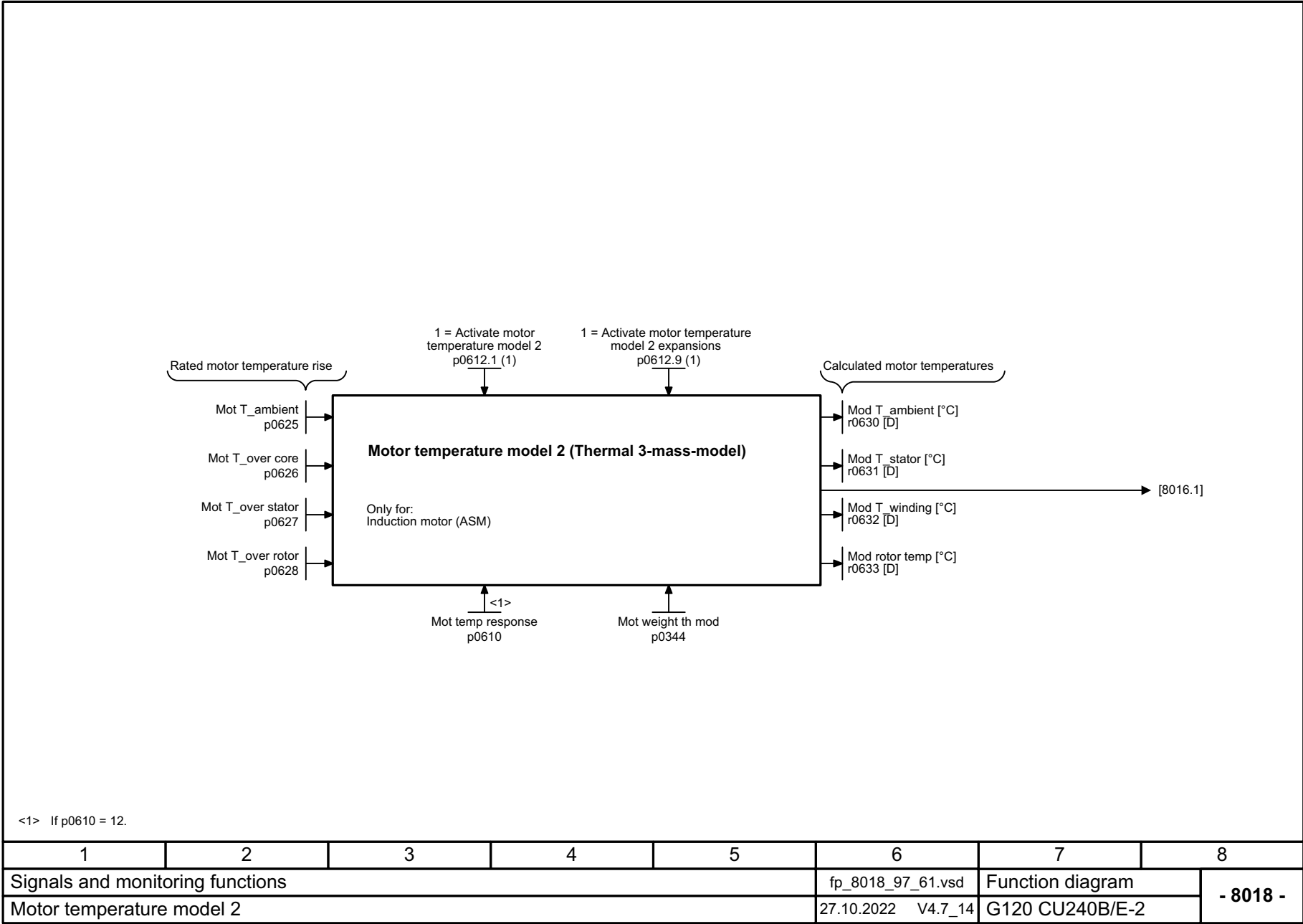
图 3-177 8018 - 电机温度模型 2
