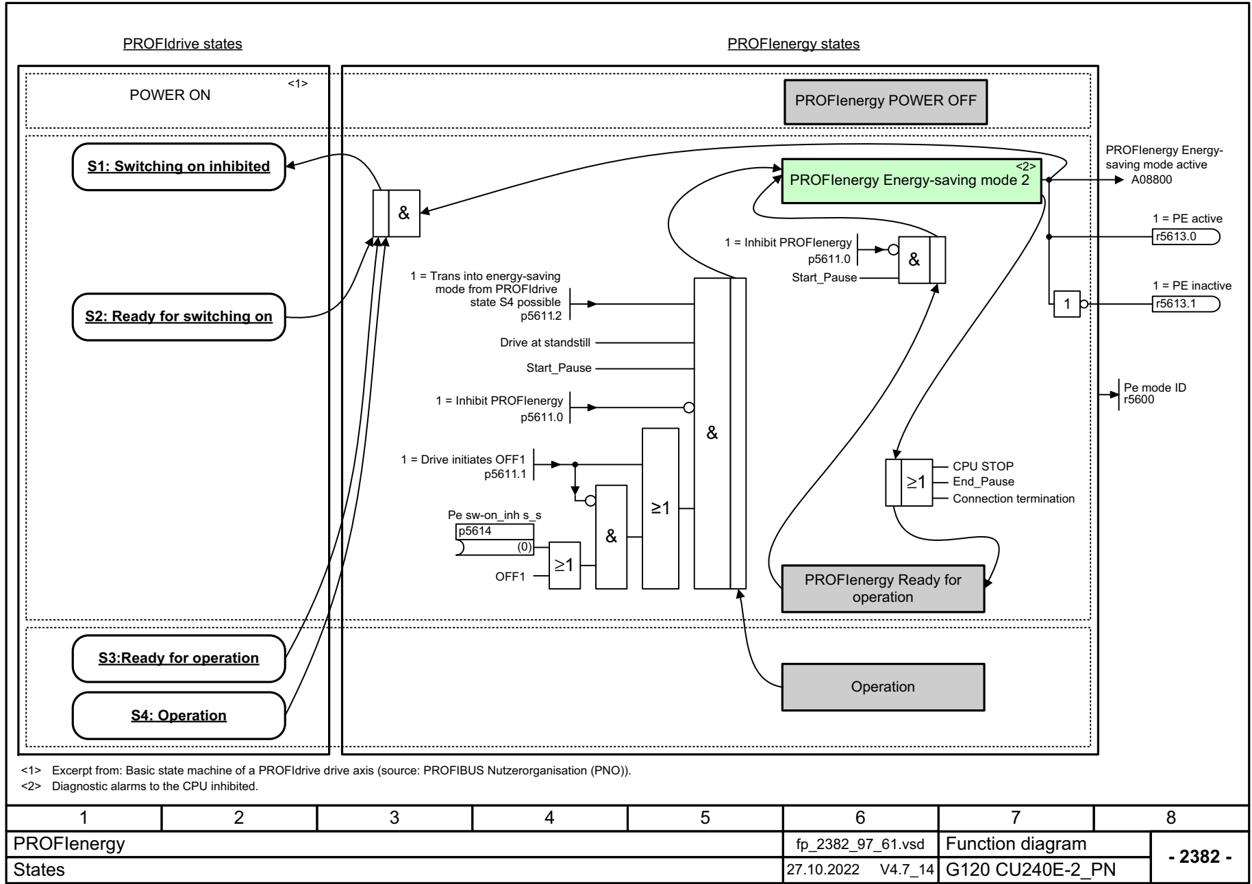
图 3-20 2382 - 状态
