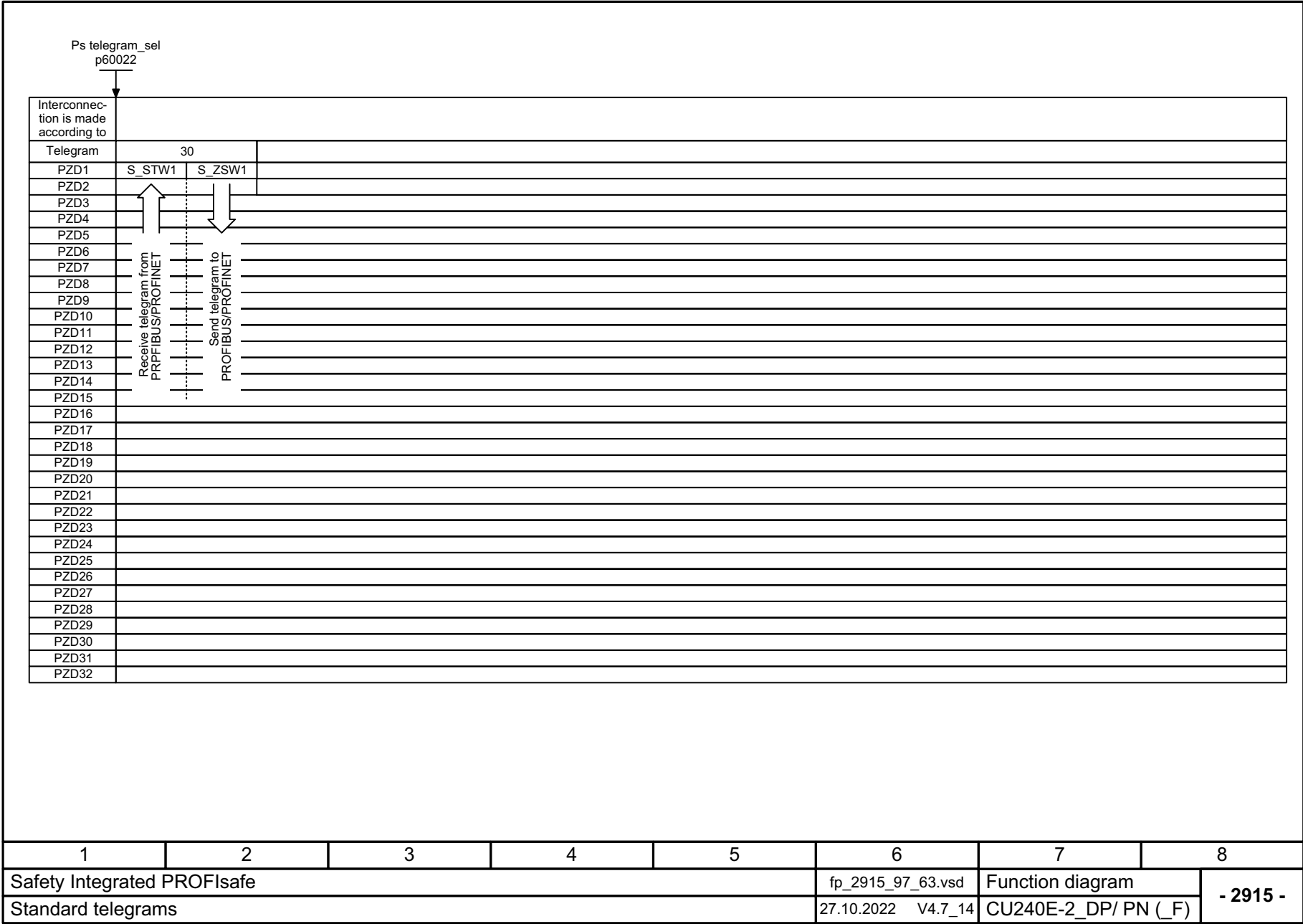
图 3-76 2915 - 标准报文
