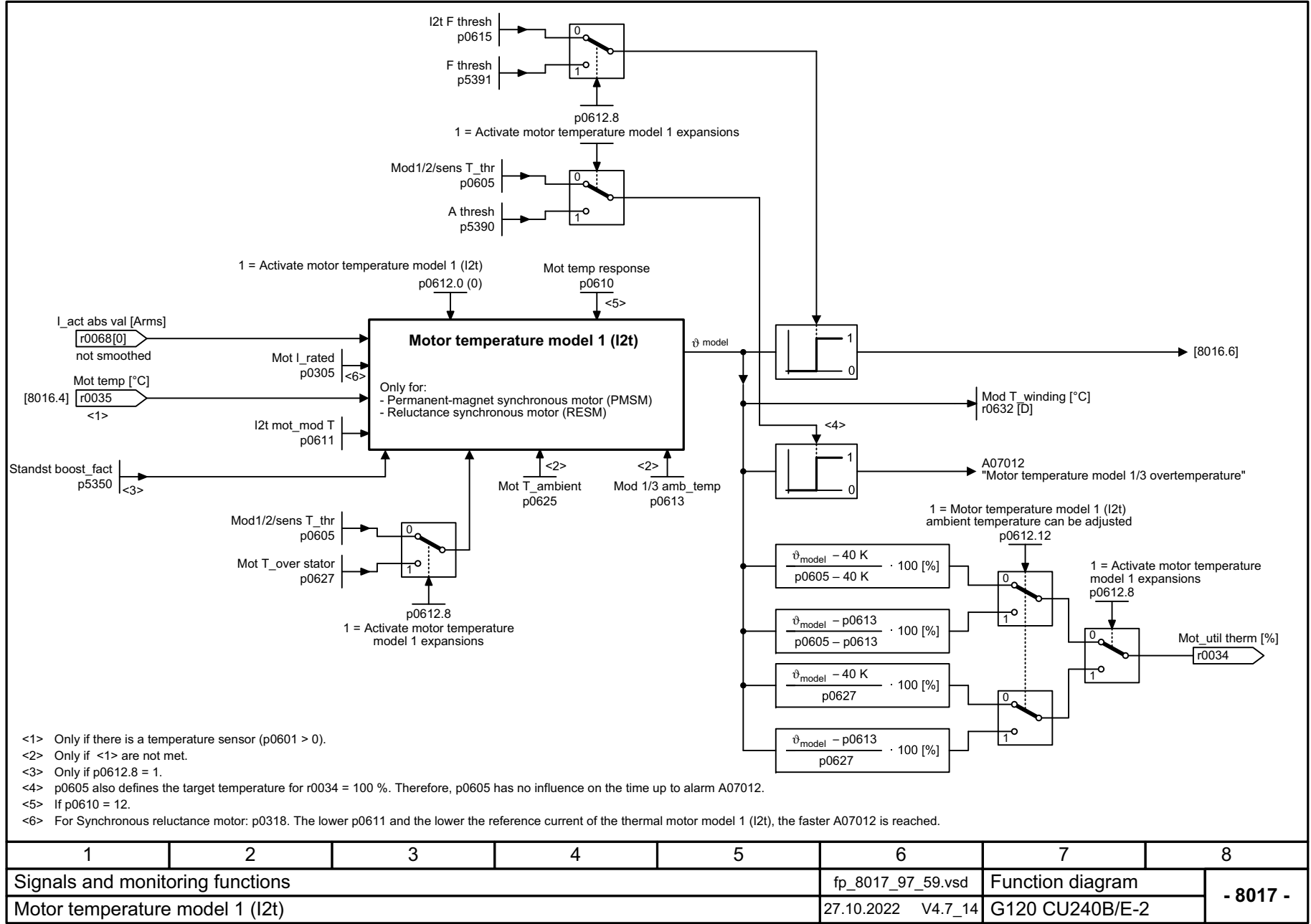
图 3-176 8017 - 电机温度模型 1 (I2t)
