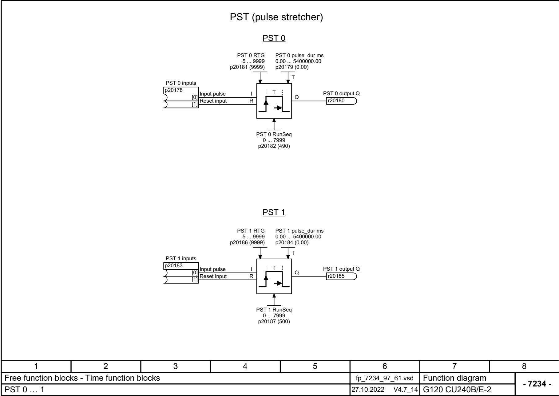
图 3-157 7234 - PST 0 ... 1
