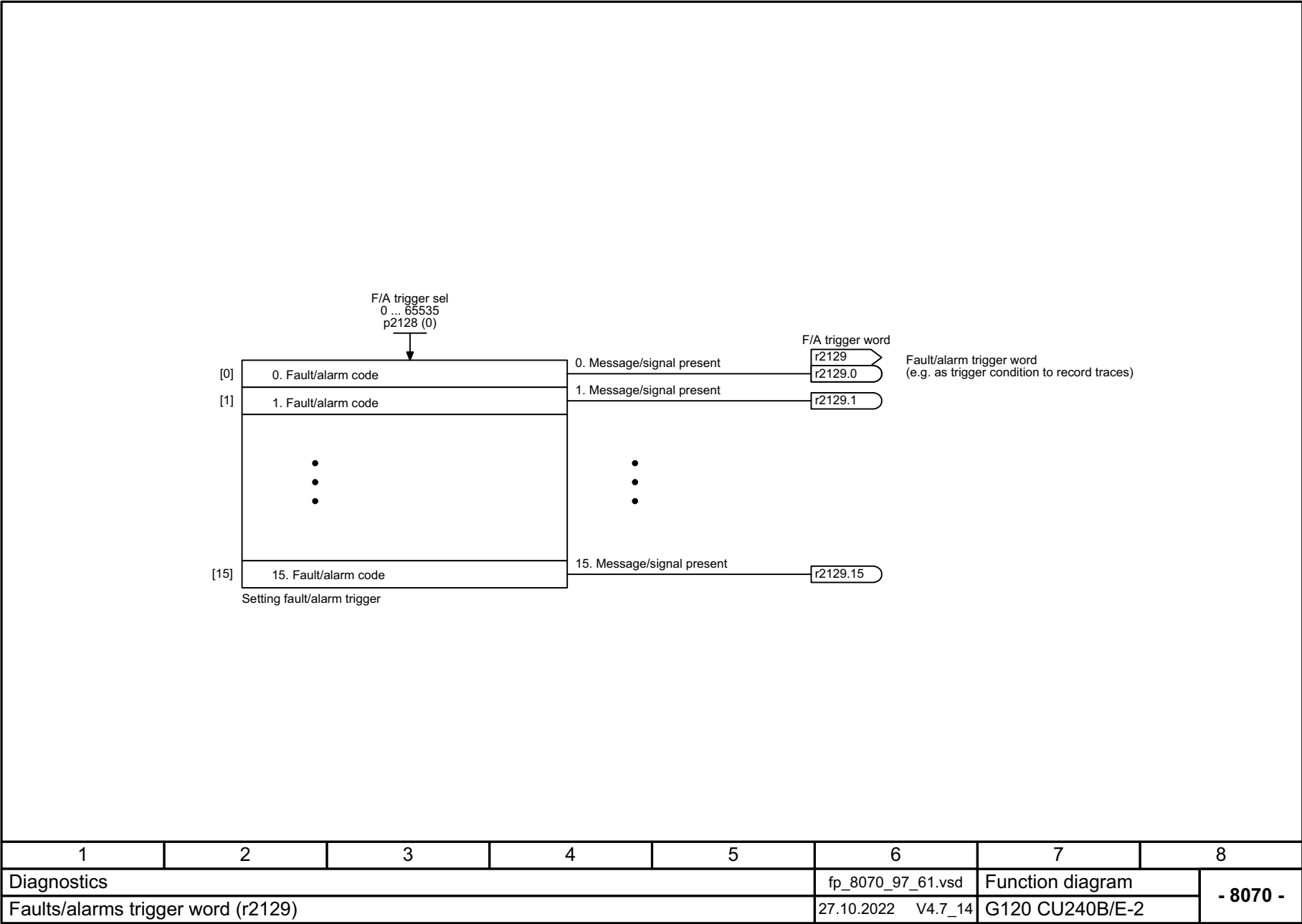
图 3-185 8070 - 故障 / 报警触发字 (r2129)
