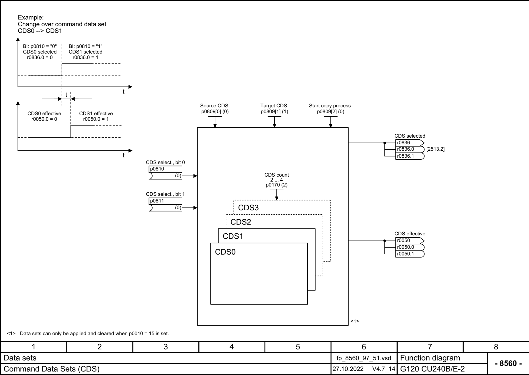
图 3-187 8560 - 指令数据组 (Command Data Set, CDS)
