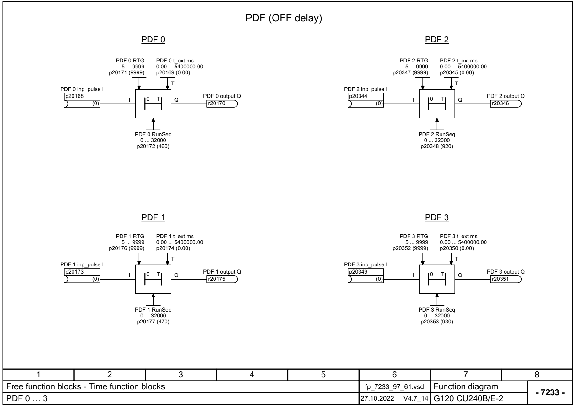
图 3-156 7233 - PDF 0 ... 3
