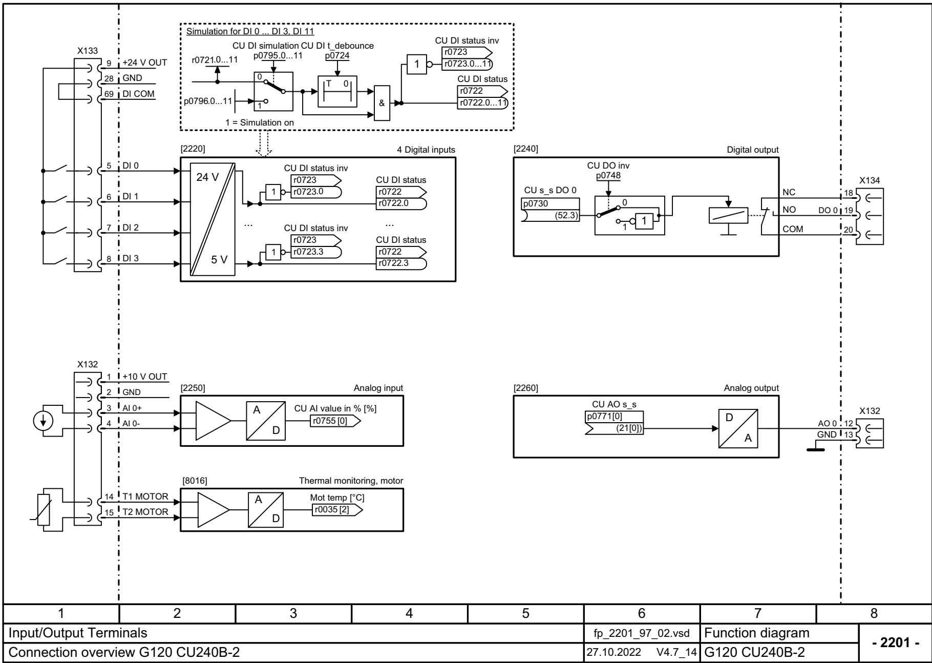
图 3-5 2201 - 接口一览 G120 CU240B-2
