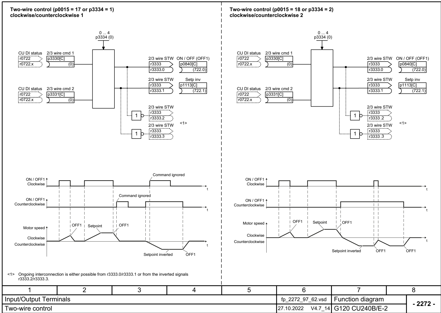
图 3-17 2272 - 双线圈控制
