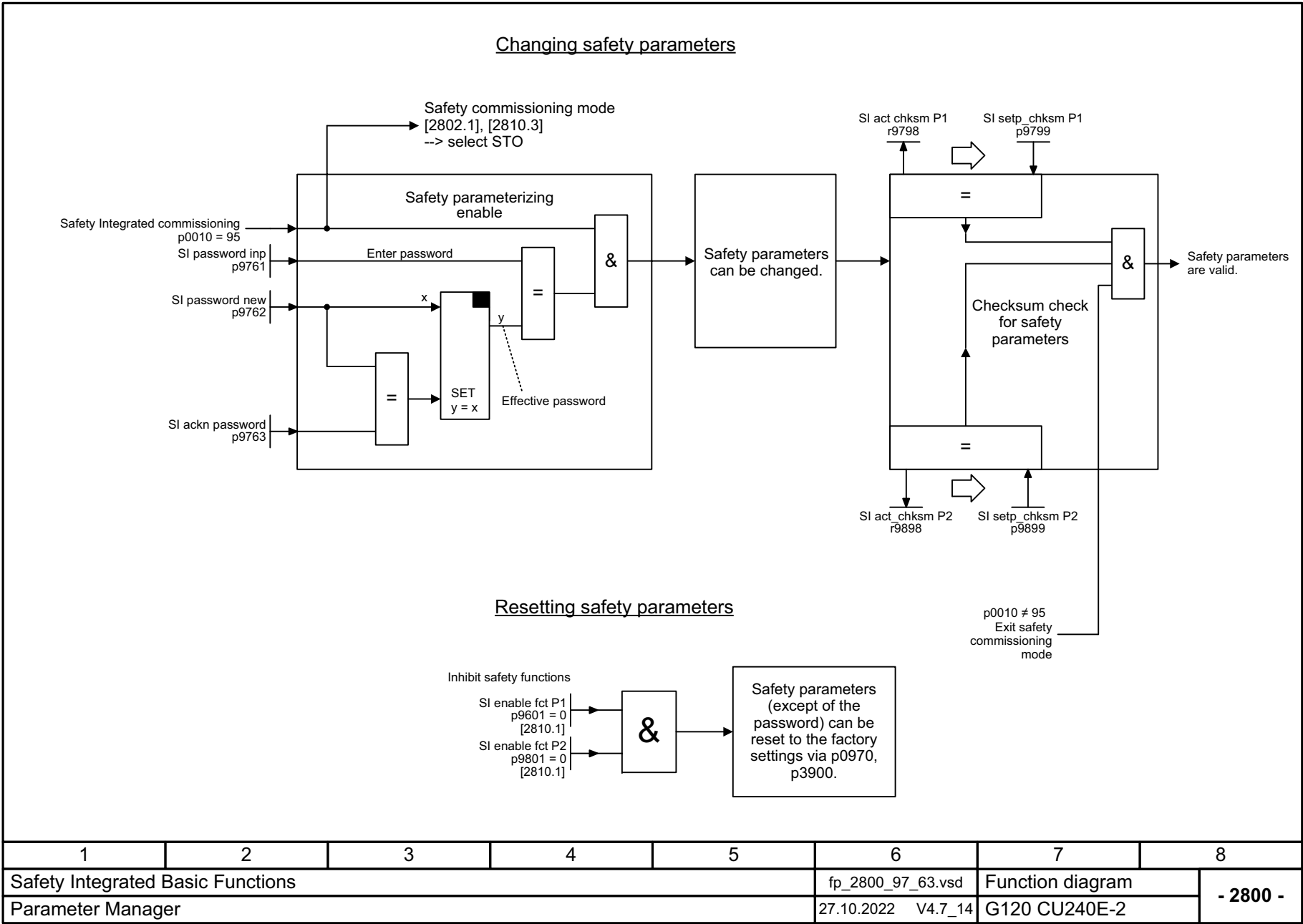
图 3-61 2800 - 参数管理器
