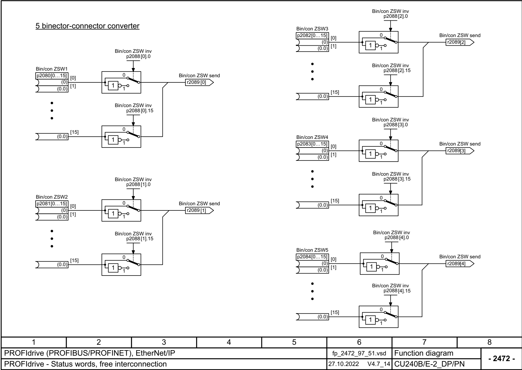
图 3-34 2472 - PROFIdrive - 自由互联状态字
