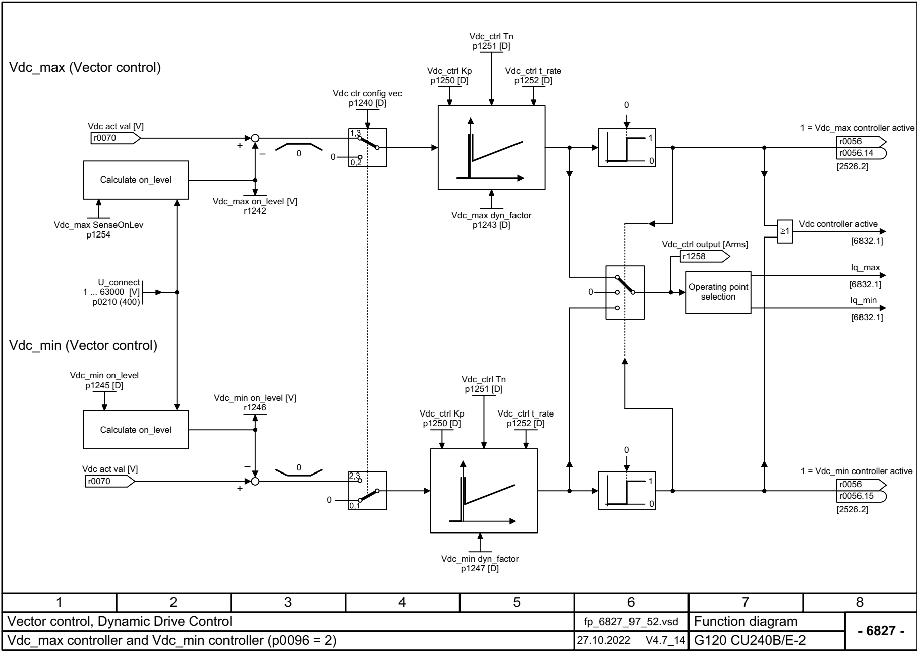
图 3-129 6827 - Vdc_max 控制器和 Vdc_min 控制器 (p0096 = 2)
