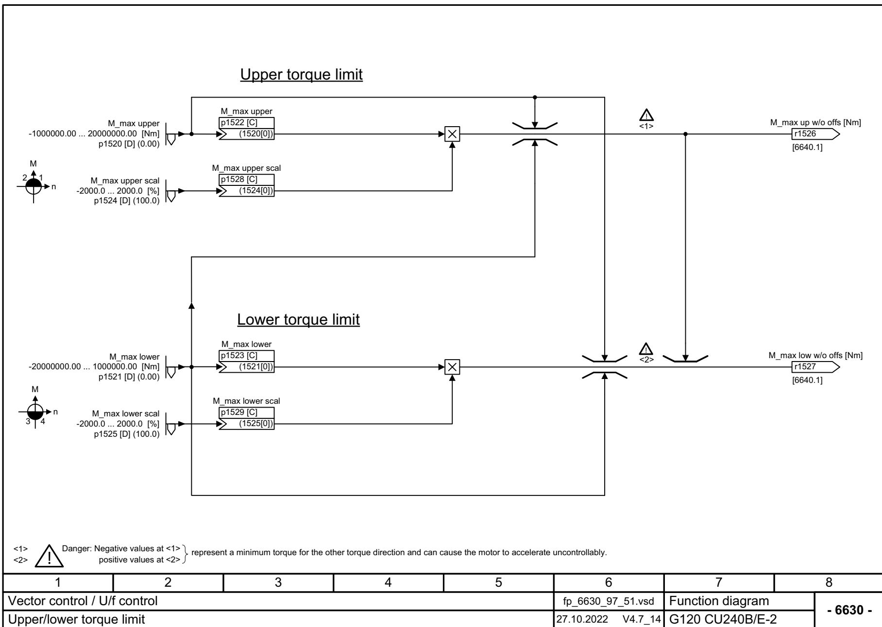
6630 - 转矩上限 / 转矩下限
