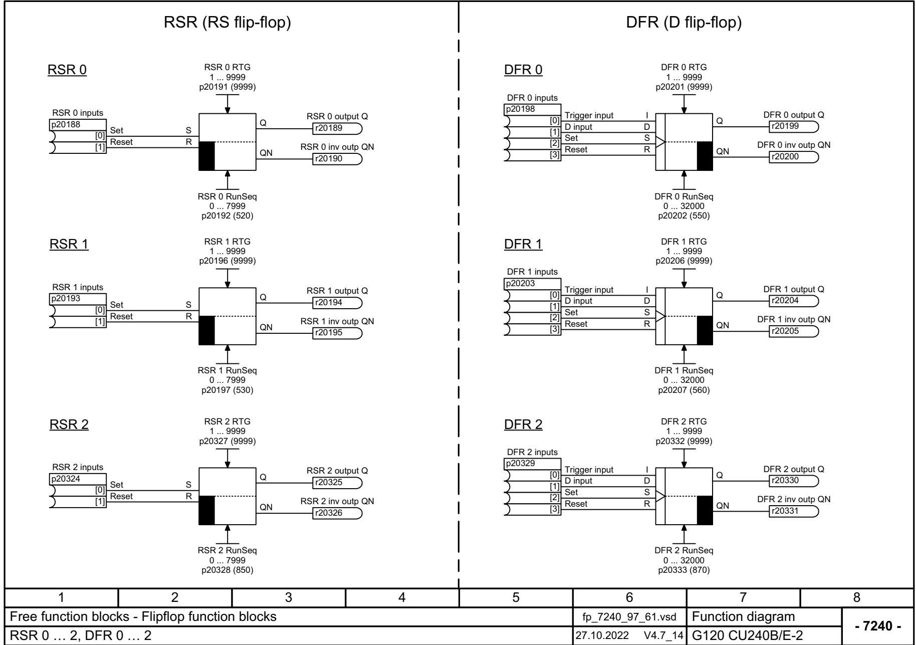
图 3-158 7240 - RSR 0 ... 2, DFR 0 ... 2
