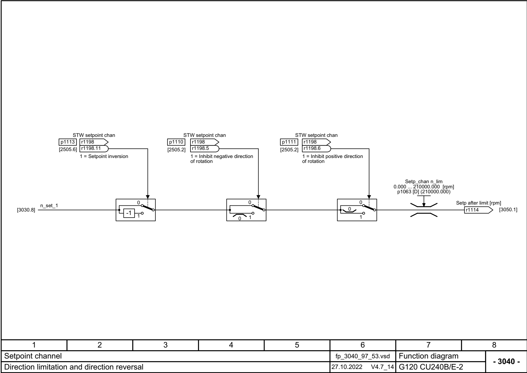
图 3-83 3040 - 方向限制和换向
