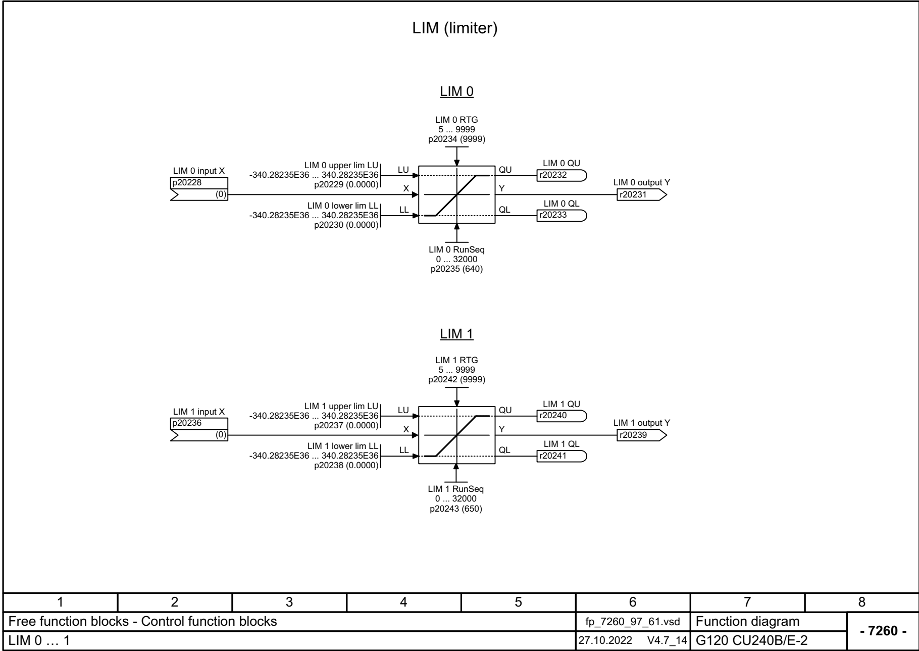
图 3-160 7260 - LIM 0 ... 1
