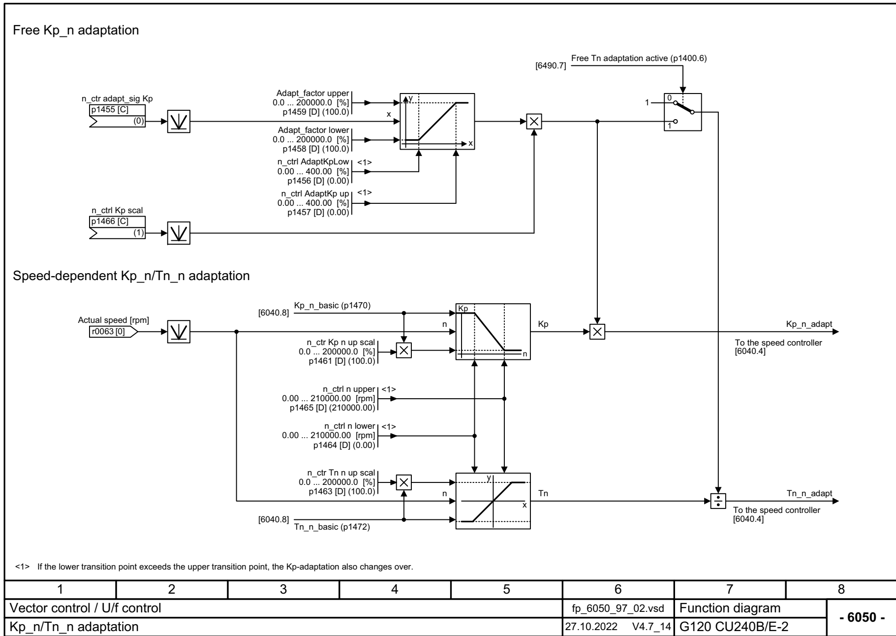
图 3-94 6050 - Kp_n-/Tn_n 适配
