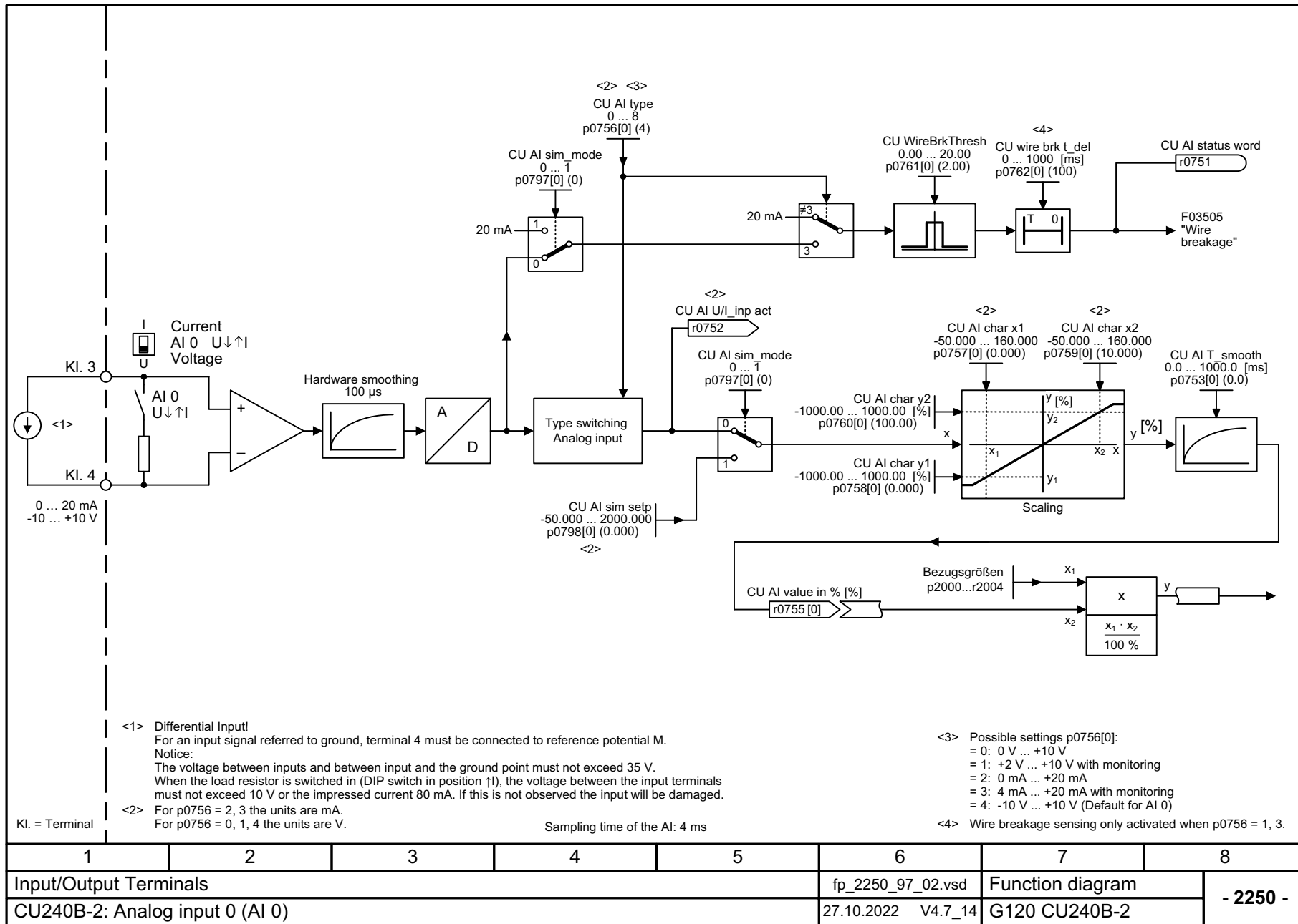
图 3-11 2250 - CU240B-2: 模拟量输入 0 (AI 0)
