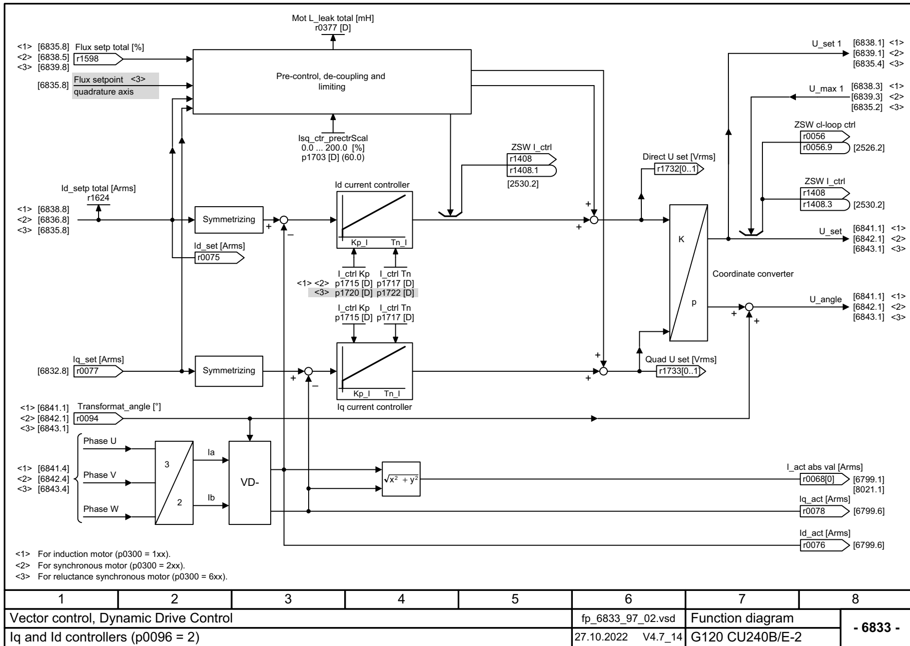
图 3-132 6833 - Iq 控制器和 Id 控制器 (p0096 = 2)
