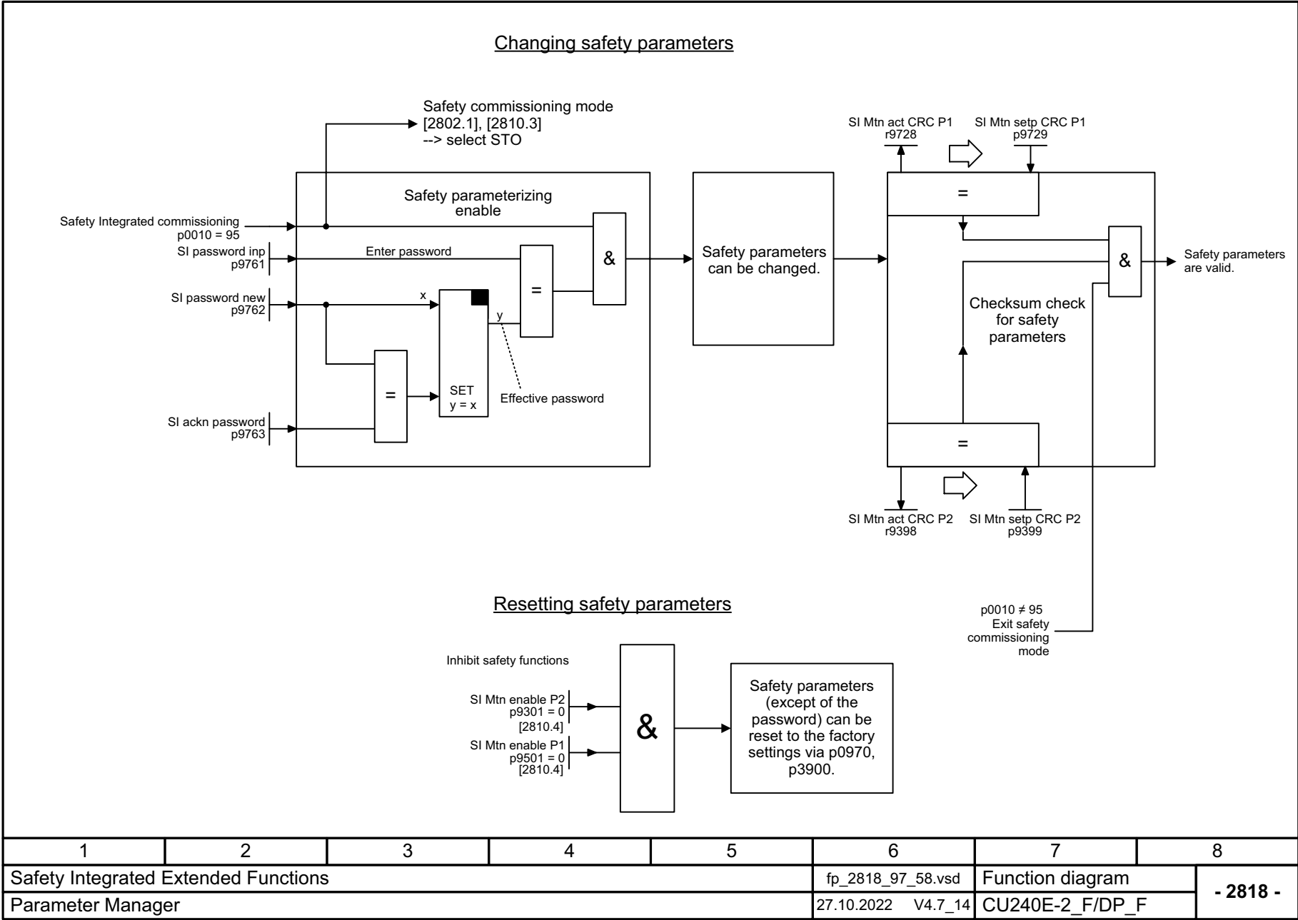
图 3-67 2818 - 参数管理器
