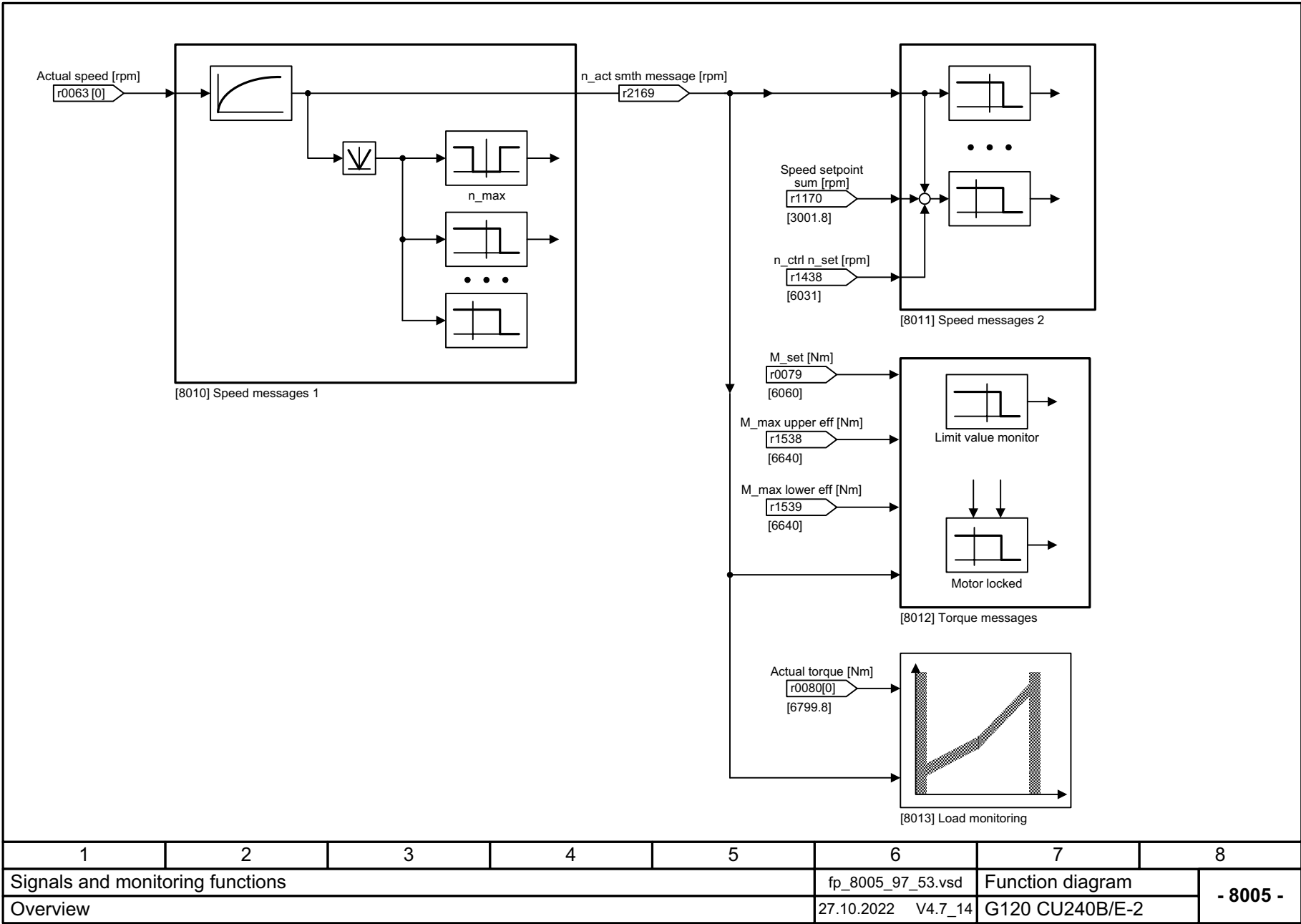
图 3-169 8005 - 一览
