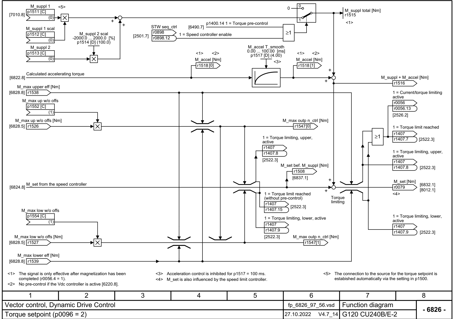
图 3-128 6826 - 转矩设定值 (p0096 = 2)
