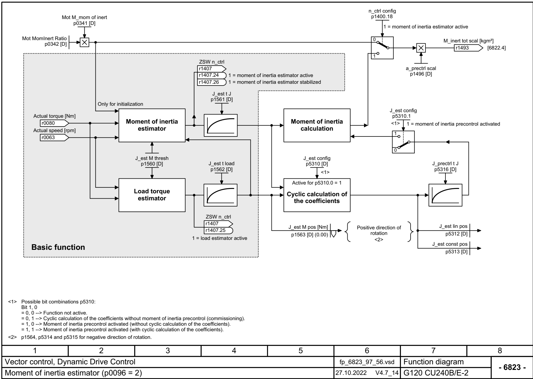
图 3-126 6823 - 转动惯量估算器 (p0096 = 2)
