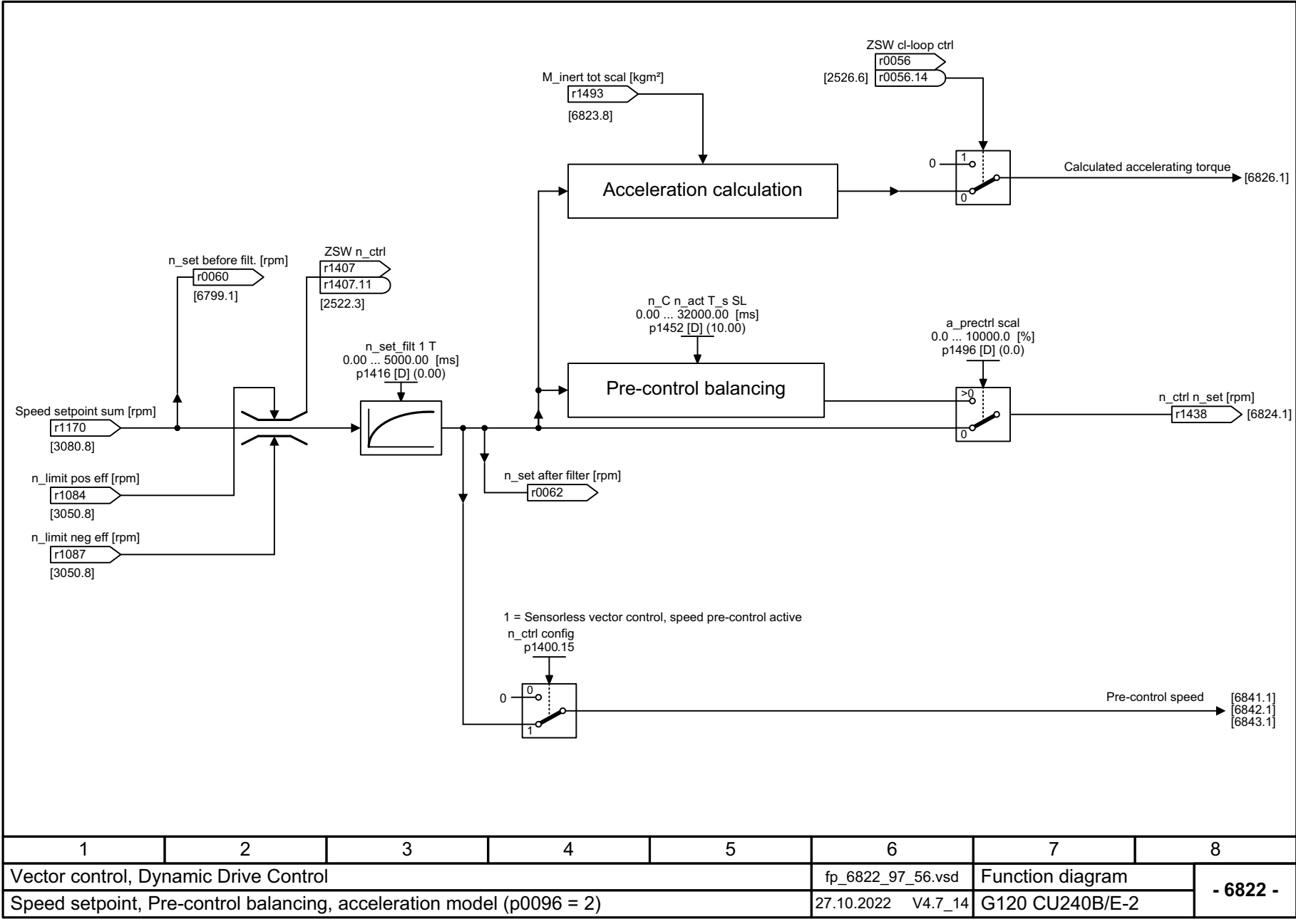
图 3-125 6822 - 转速设定值, 前馈对称性, 加速度模型 (p0096 = 2)
