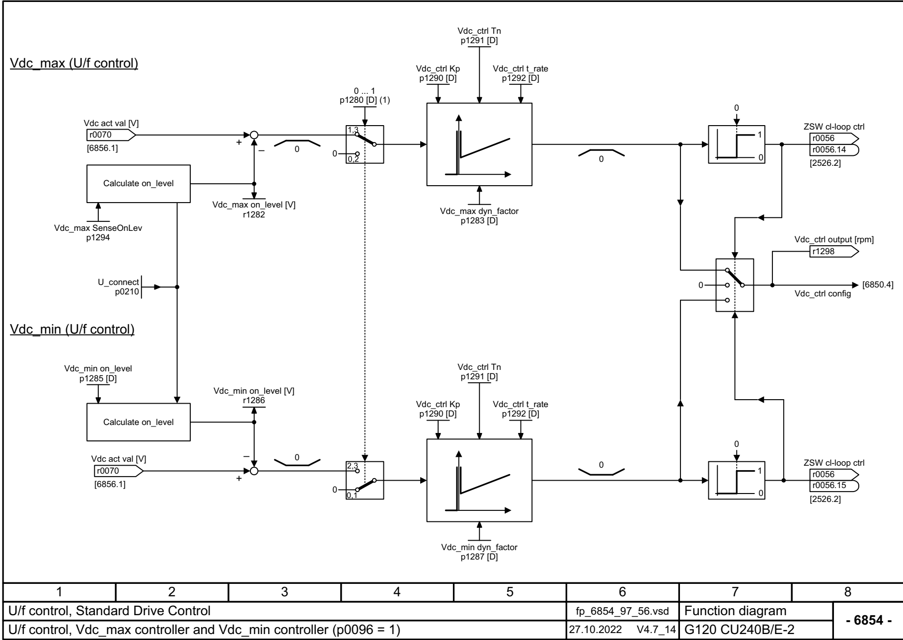
图 3-121 6854 - V/f 控制、Vdc_max 控制器和 Vdc_min 控制器 (V/f) (p0096=1)
