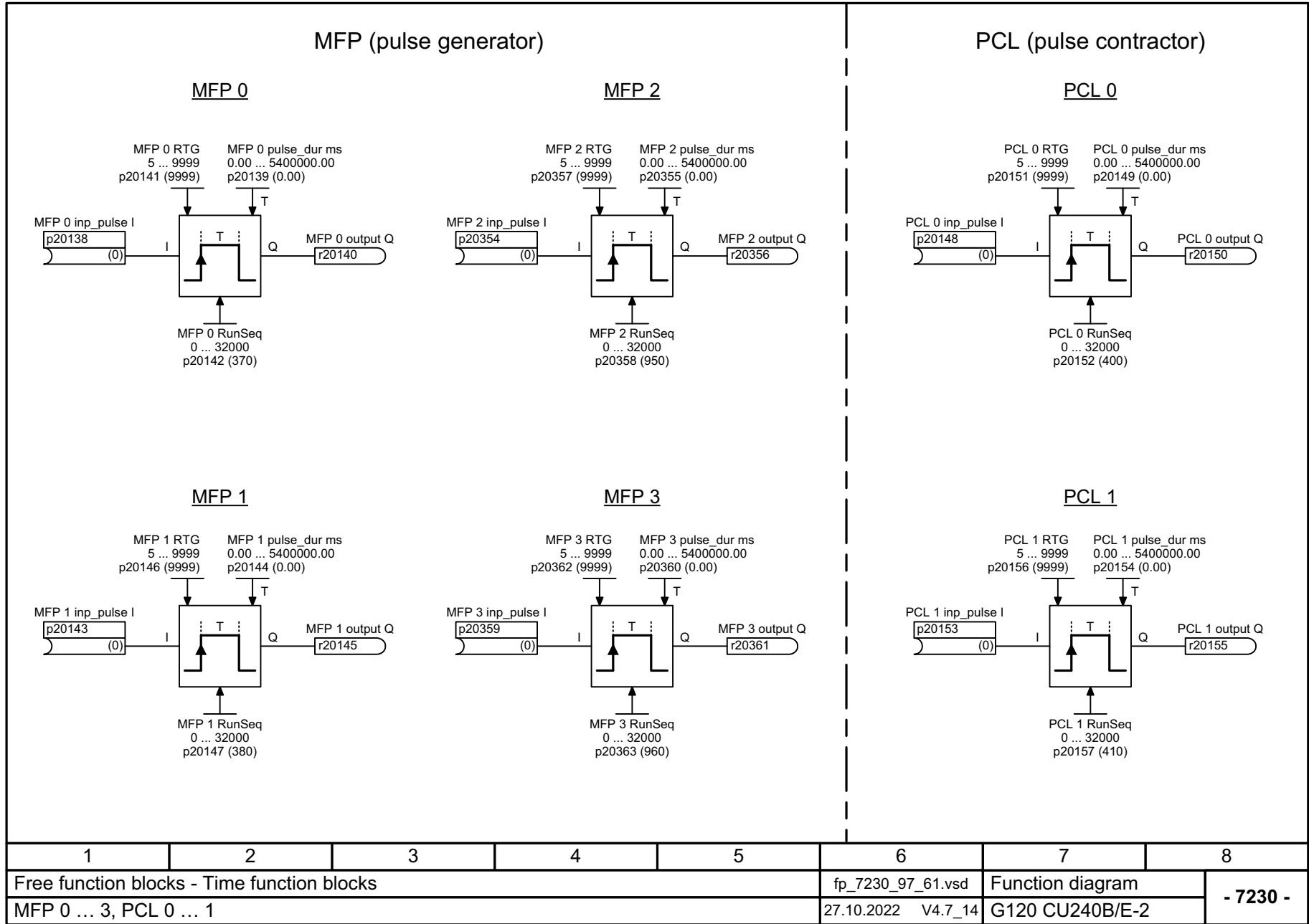
图 3-154 7230 - MFP 0 ... 3, PCL 0 ... 1
