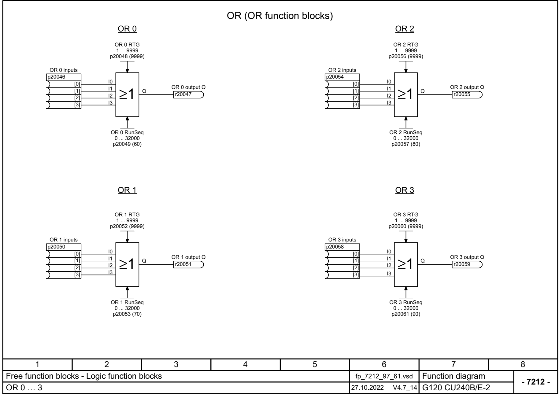
图 3-146 7212 - OR 0 ... 3
