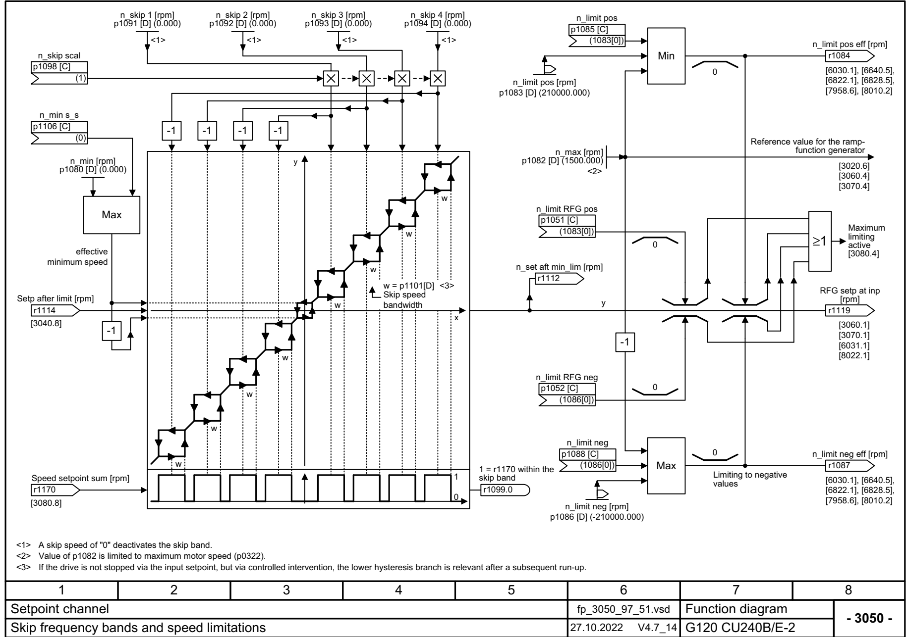
图 3-84 3050 - 跳转频带和转速限制
