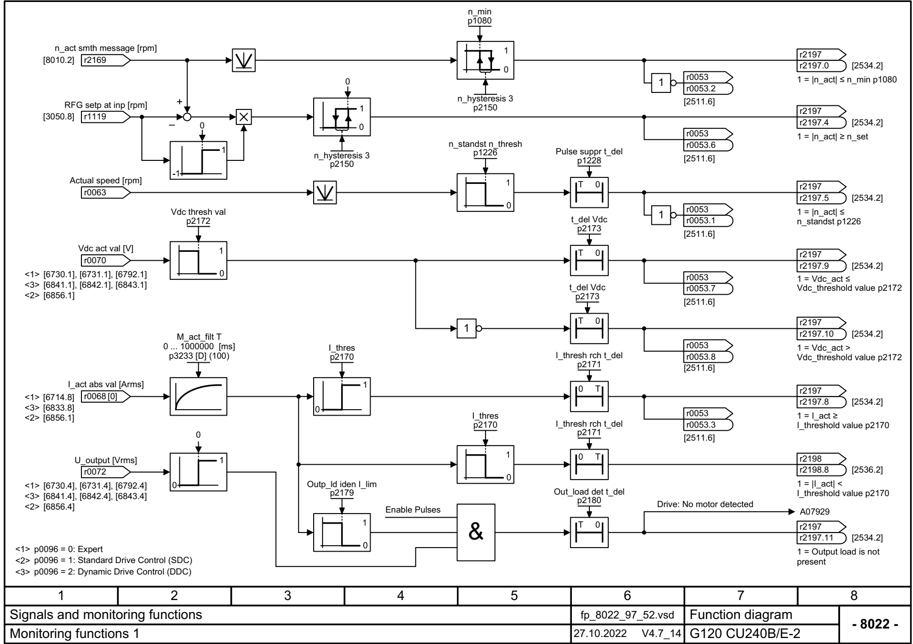
图 3-180 8022 - 监控功能 1
