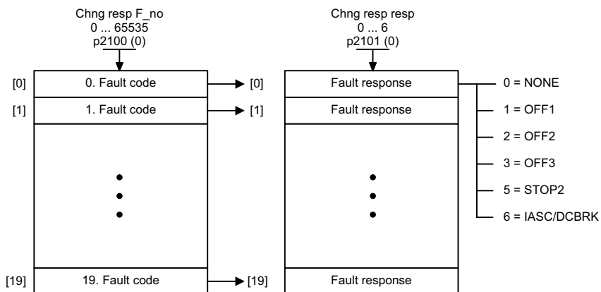
图 3-186 8075 - 故障 / 报警配置
