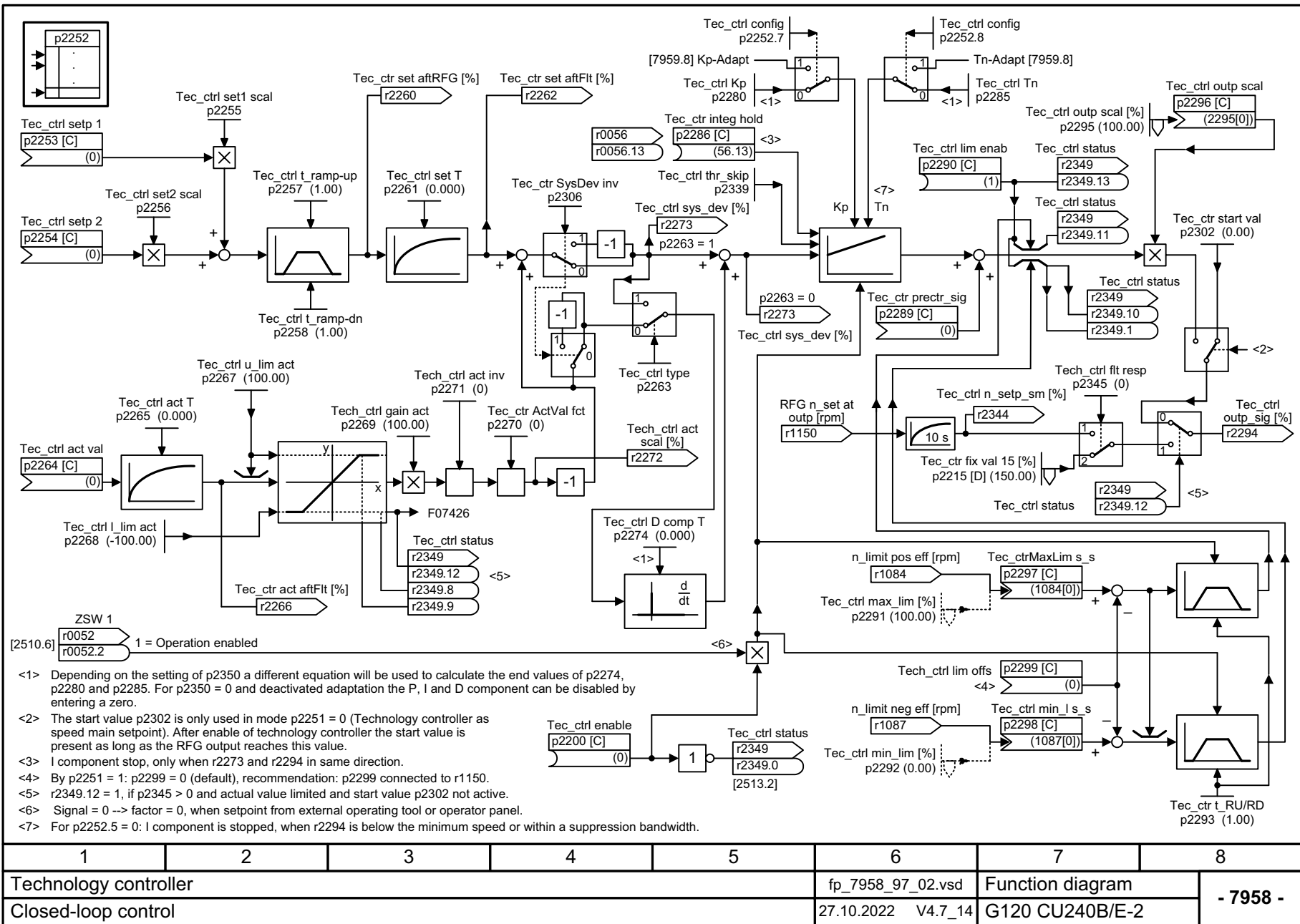
图 3-167 7958 - 闭环控制
