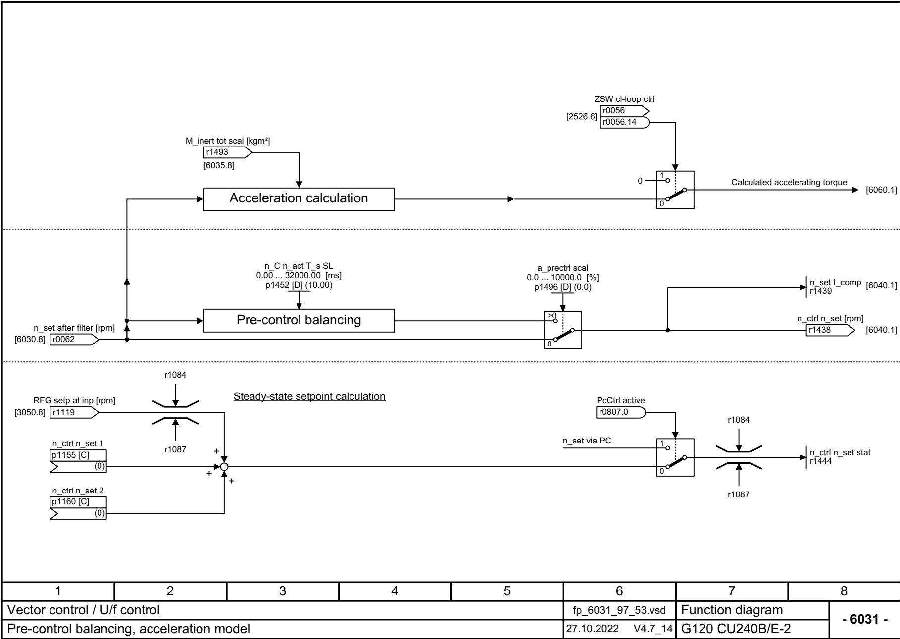
图 3-91 6031 - 前馈对称性, 加速度模型
