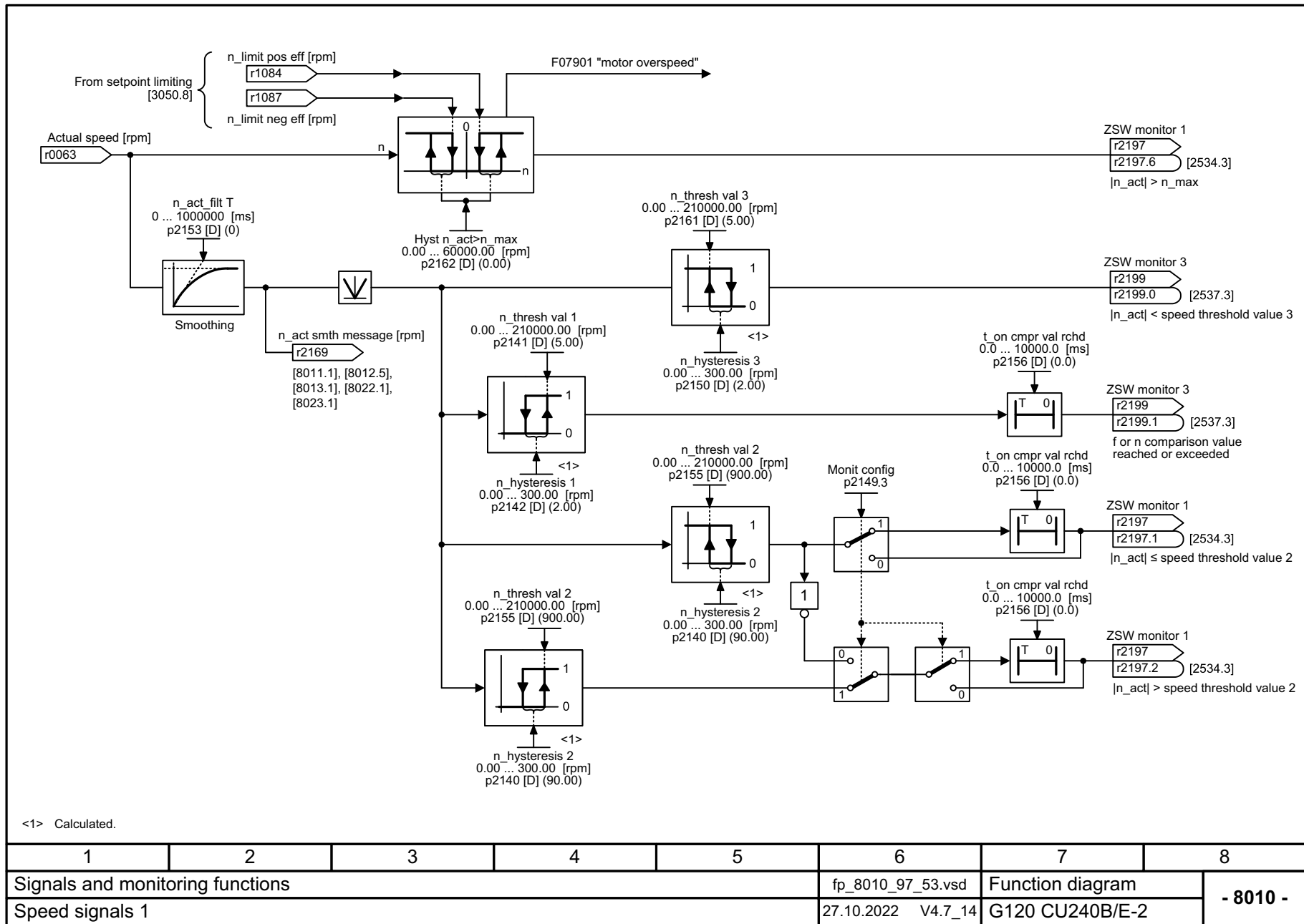
图 3-170 8010 - 转速信息 1
