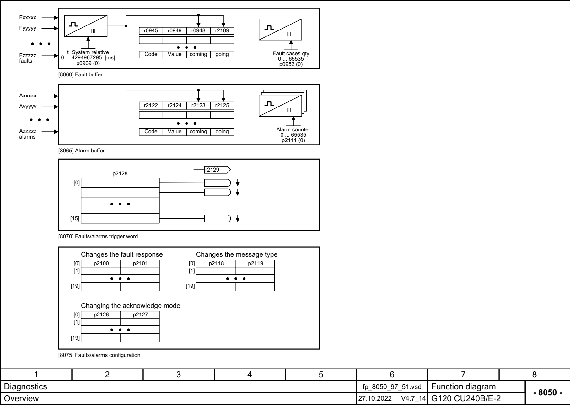
图 3-182 8050 - 一览
