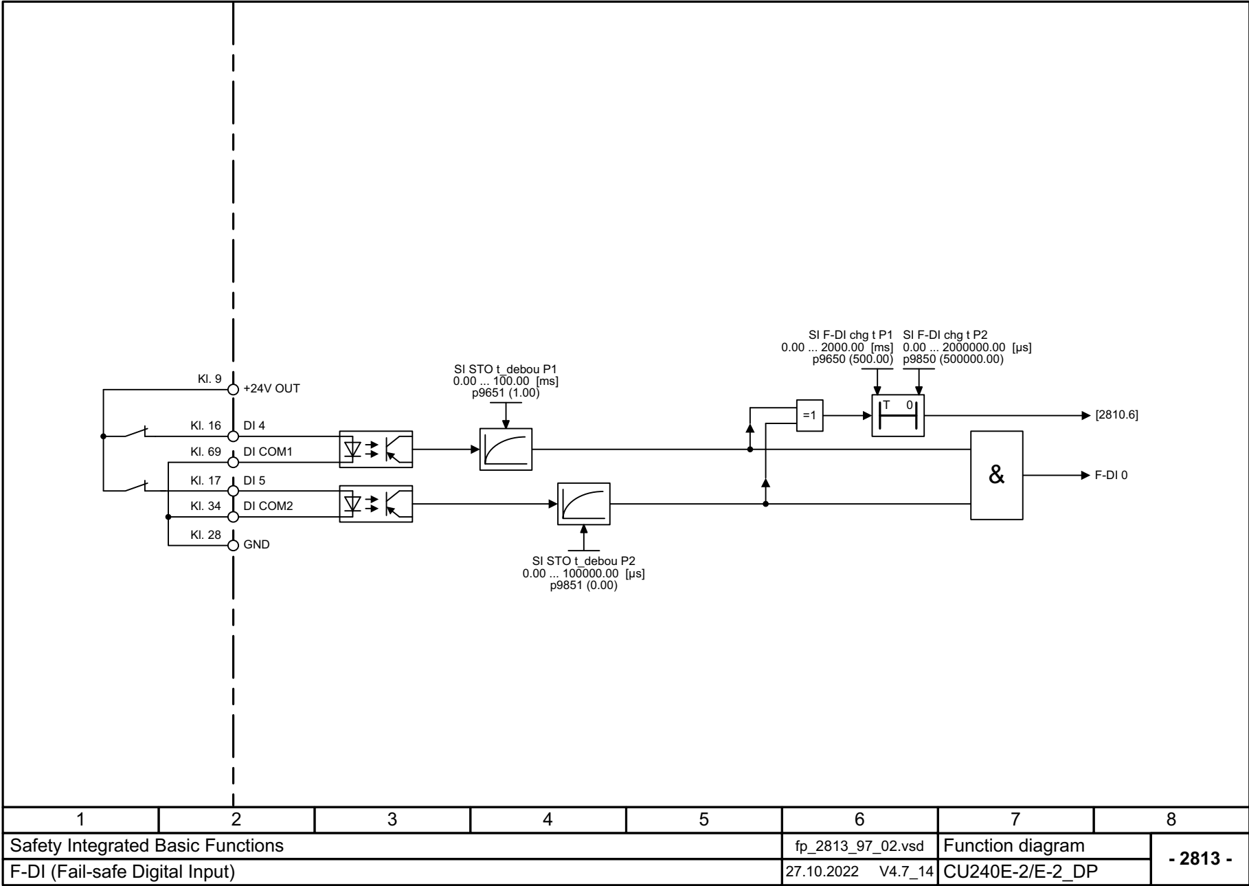
图 3-66 2813 - F-DI (Fail-safe Digital Input)
