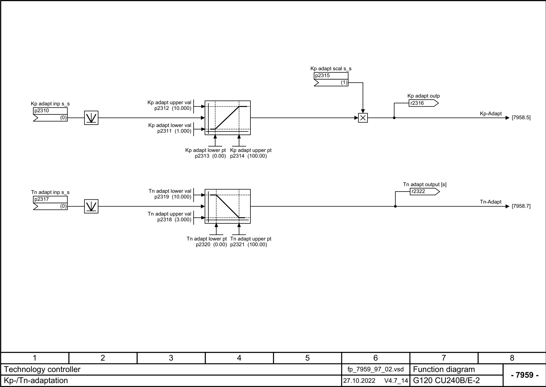
图 3-168 7959 - Kp/Tn 适配
