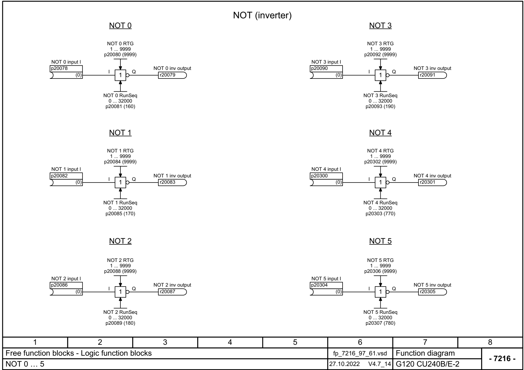
图 3-148 7216 - NOT 0 ... 5
