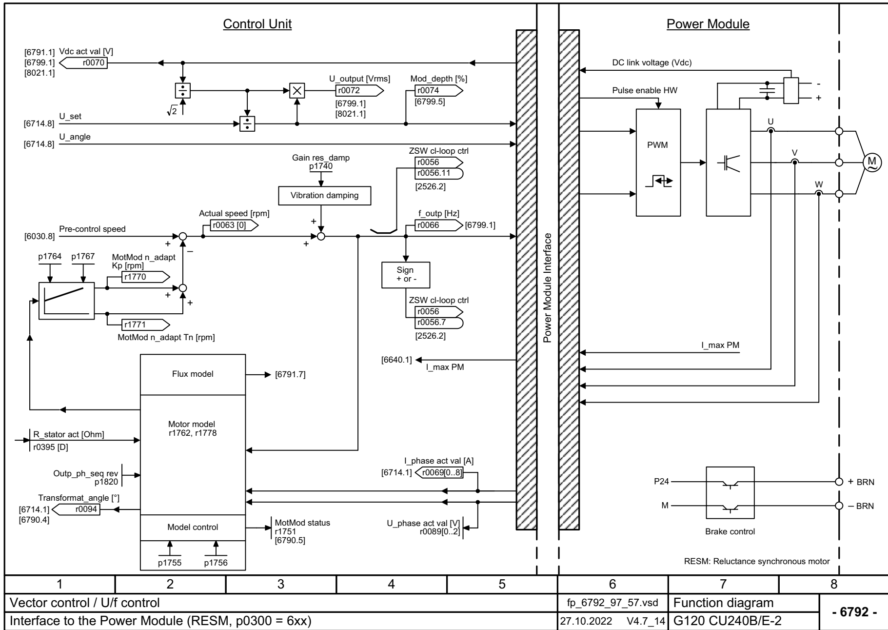
图 3-116 6792 - 和功率模块的接口 (RESM, p0300 = 6xx)
