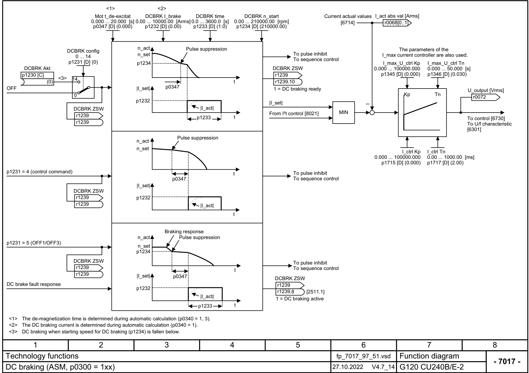
图 3-143 7017 - 直流制动 (ASM, p0300 = 1)
