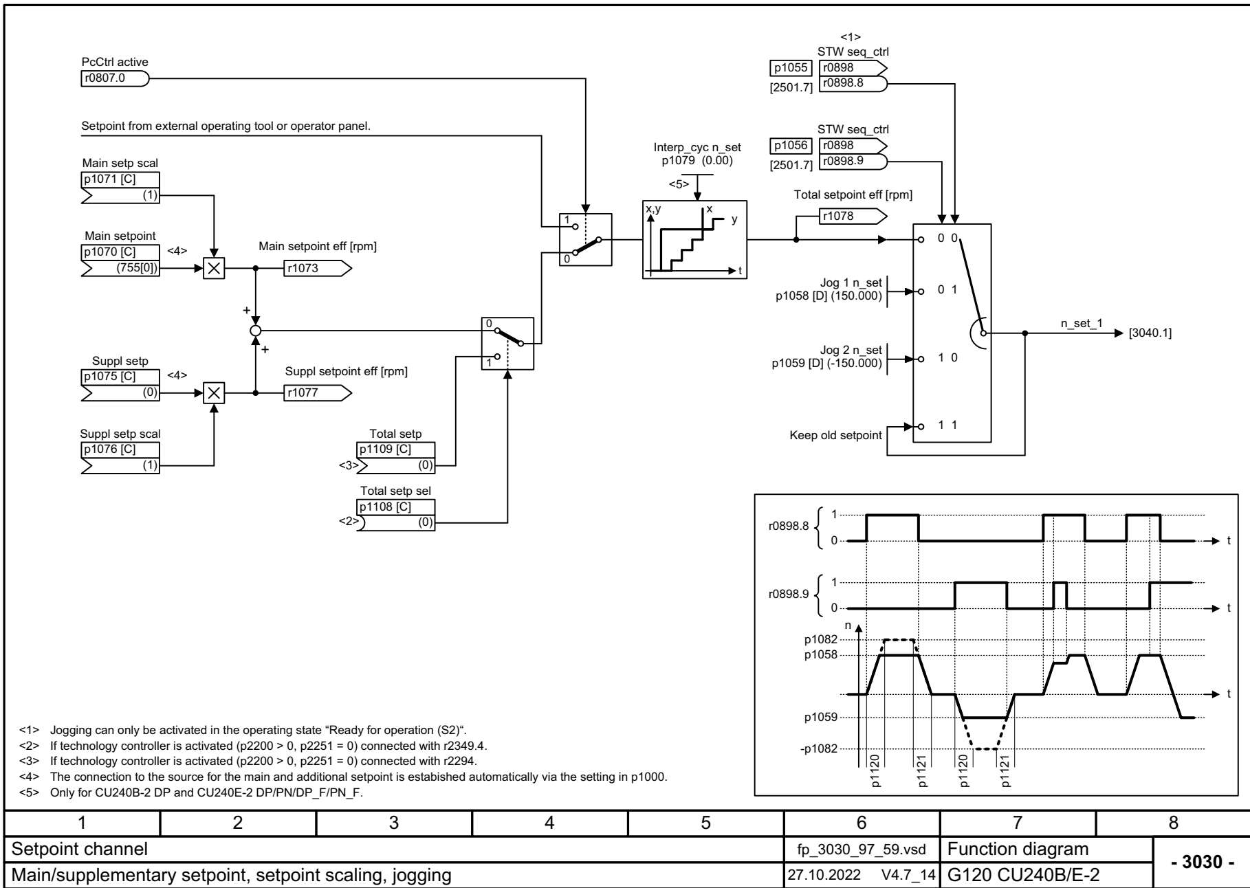
图 3-82 3030 - 主设定值 / 附加设定值，设定值比例缩放，点动
