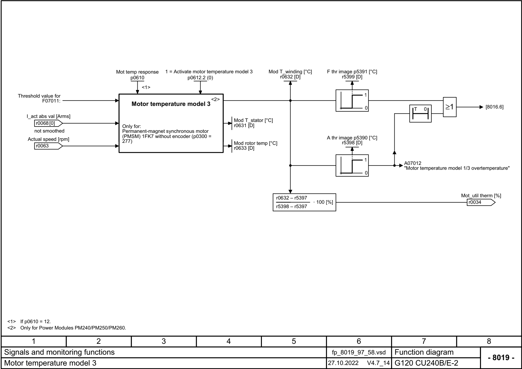
图 3-178 8019 - 电机温度模型 3
